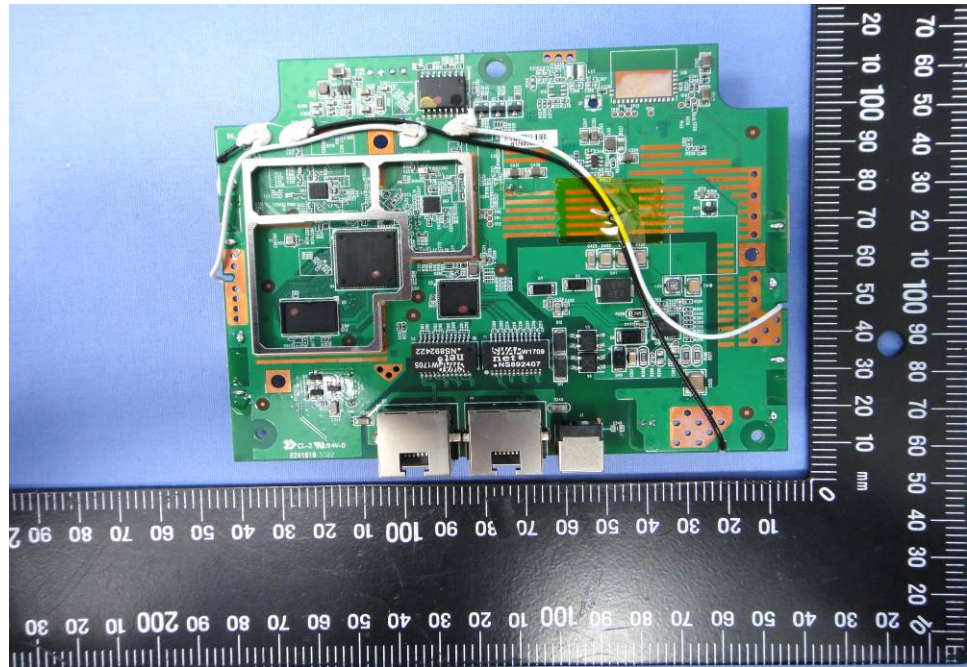
EUT Photo (14)
