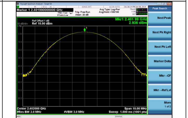
\pi/4 DQPSK-LCH
