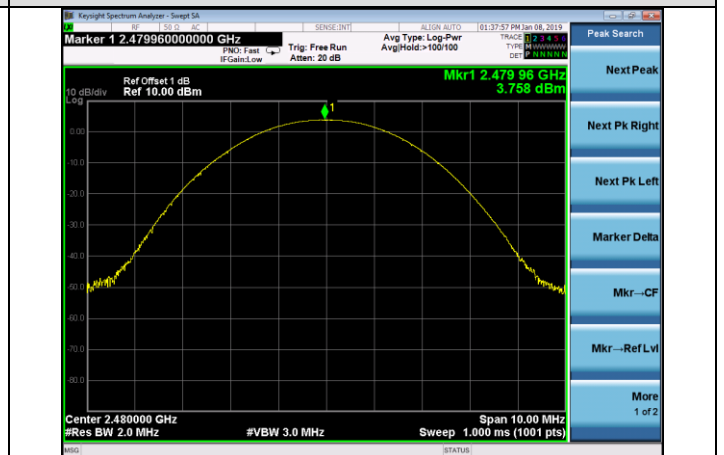
\pi/4 DQPSK-HCH
