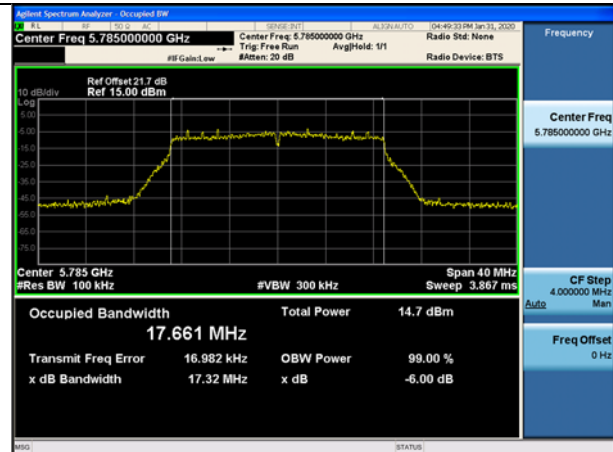
802.11ac(VHT20) (CH.157)
