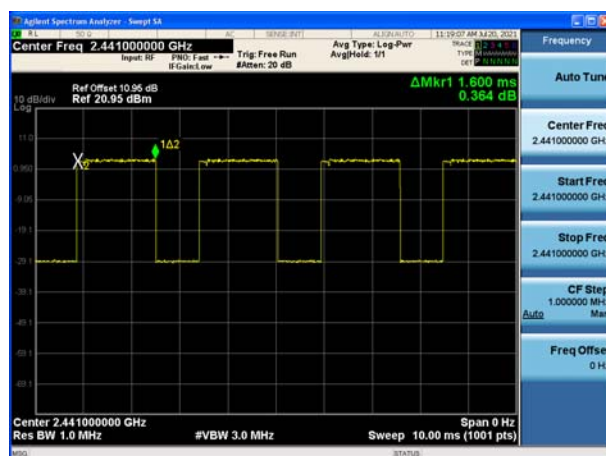
Modulation: \pi/4 DQPSK 2DH3 2441
