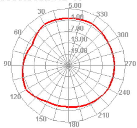
5500.000MHz H
