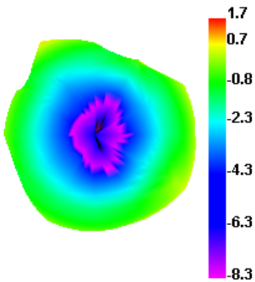
5500.000MHz E1
