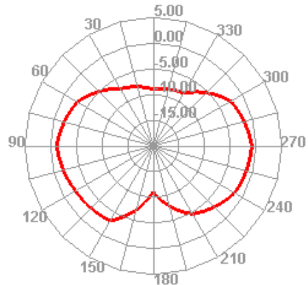
5500.000MHz E2
