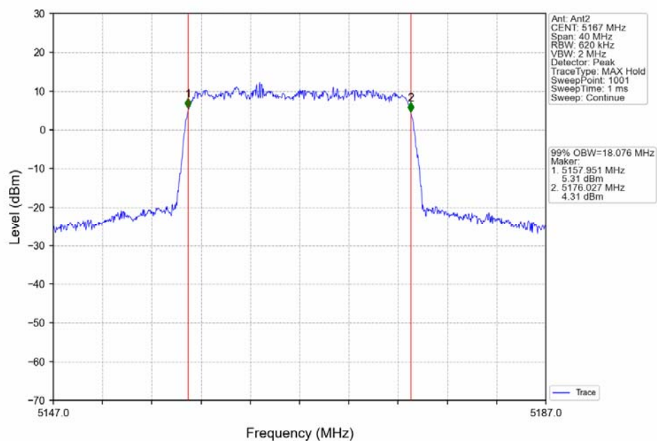
QPSK 20MHz_LCH_5167MHz_Ant2_NTNV
