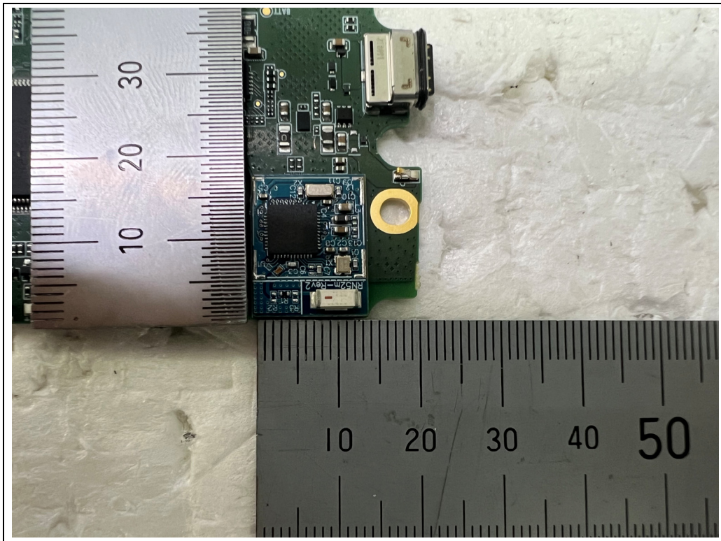
<Bluetooth LE Antenna>
