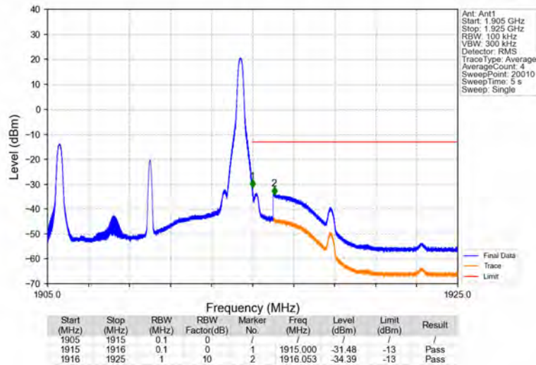
Band25_10MHz_QPSK_HCH_1910MHz_RB_1_49_NTNV
