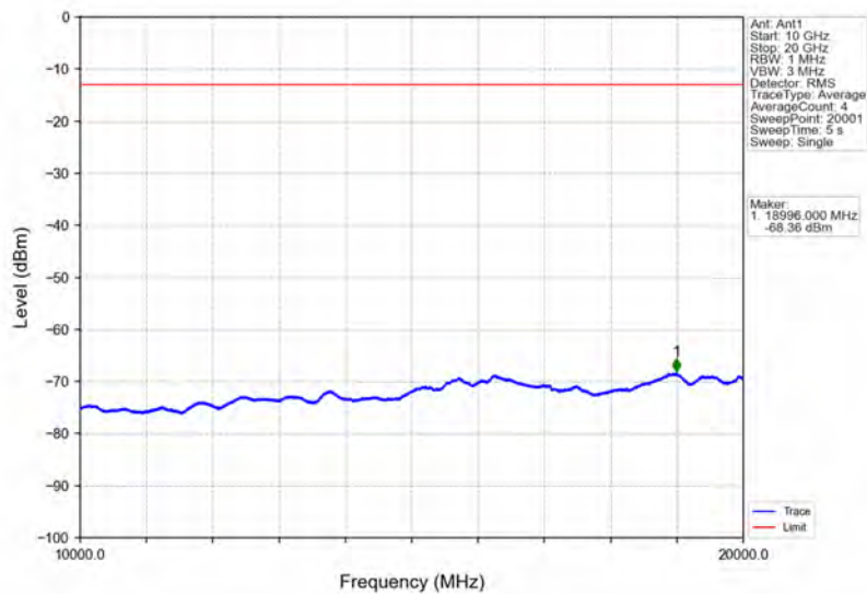
Band25_10MHz_QPSK_HCH_1910MHz_RB_1_0_NTNV
