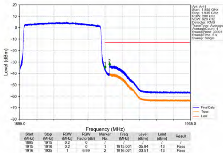
Band25_20MHz_QPSK_HCH_1905MHz_RB_100_0_NTNV
