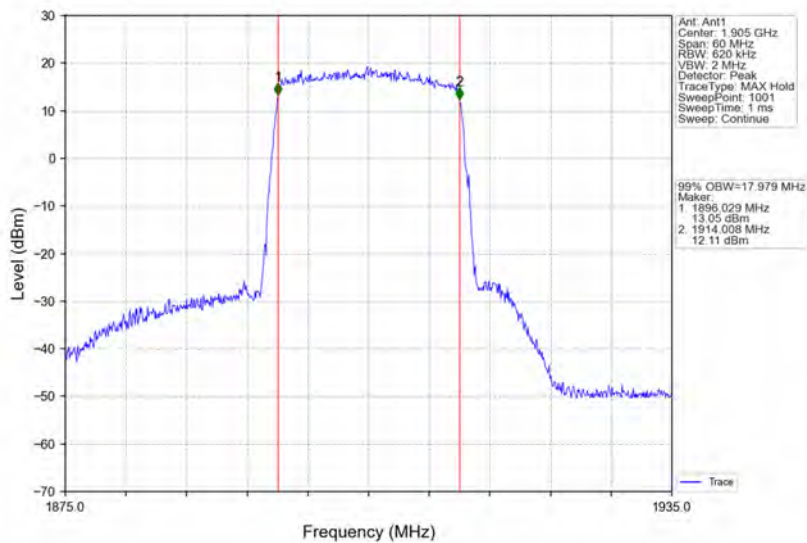
Band25_20MHz_QPSK_HCH_1905MHz_RB_100_0_NTNV
