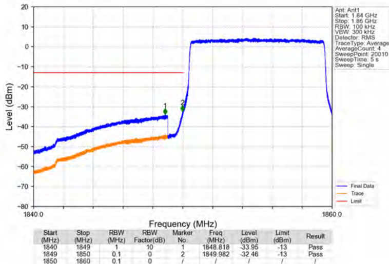
Band25_10MHz_QPSK_LCH_1855MHz_RB_50_0_NTNV
