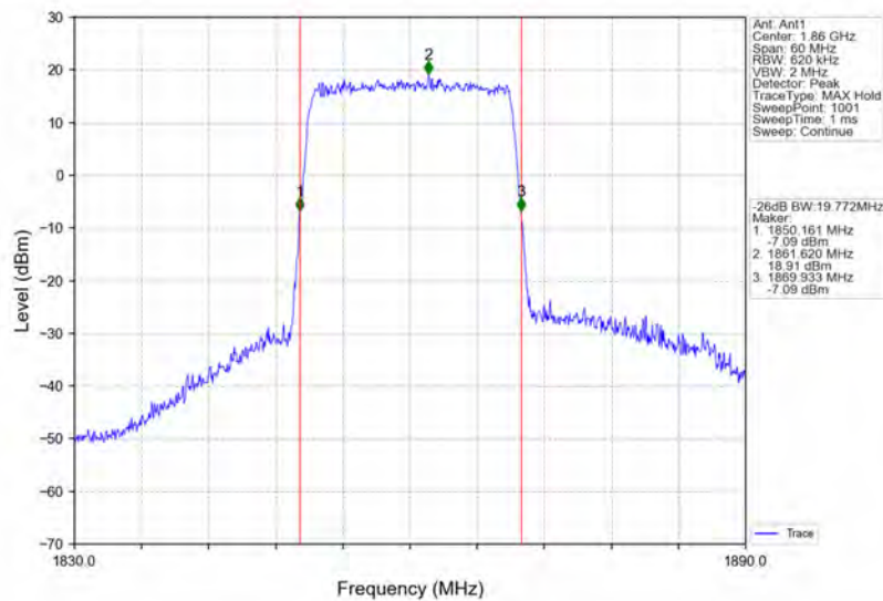
Band25_20MHz_QPSK_LCH_1860MHz_RB_100_0_NTNV
