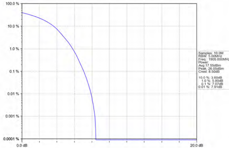
Band25_20MHz_QPSK_HCH_1905MHz_RB_100_0_NTNV
