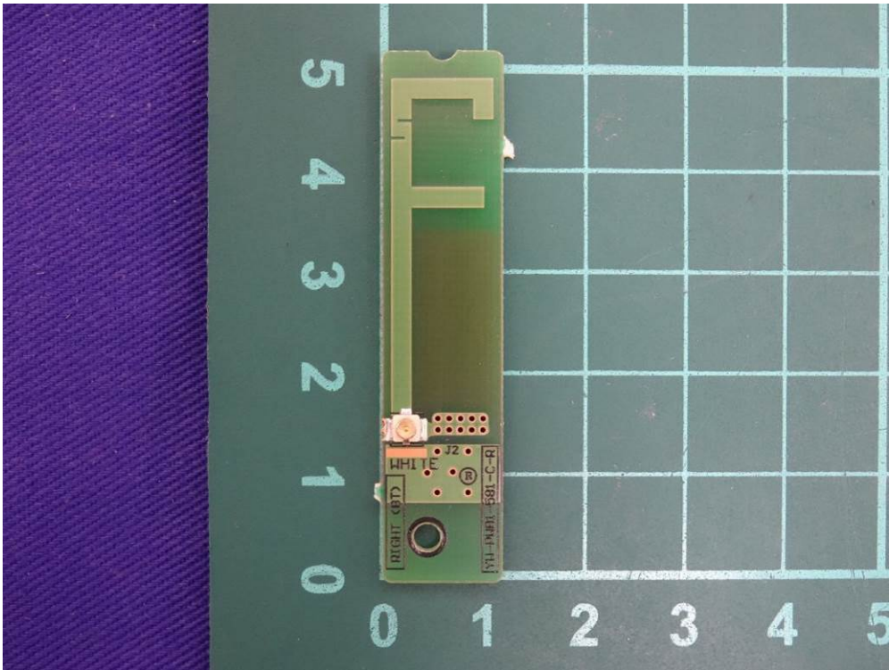
(50) EUT Photo
