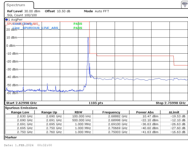
60MHz_30kHz_2659.98MHz_DFT-s-OFDM QPSK_RB1@161&-22.10 dBm
