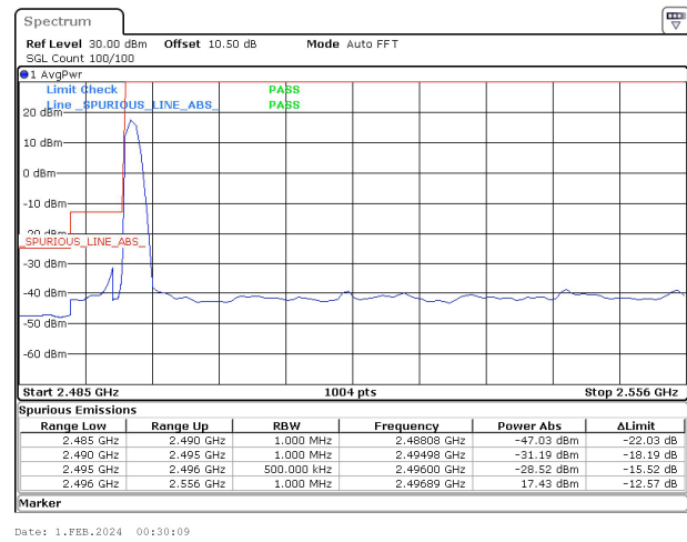
60MHz_30kHz_2526MHz_DFT-s-OFDM QPSK_RB1@0&17.43 dBm
