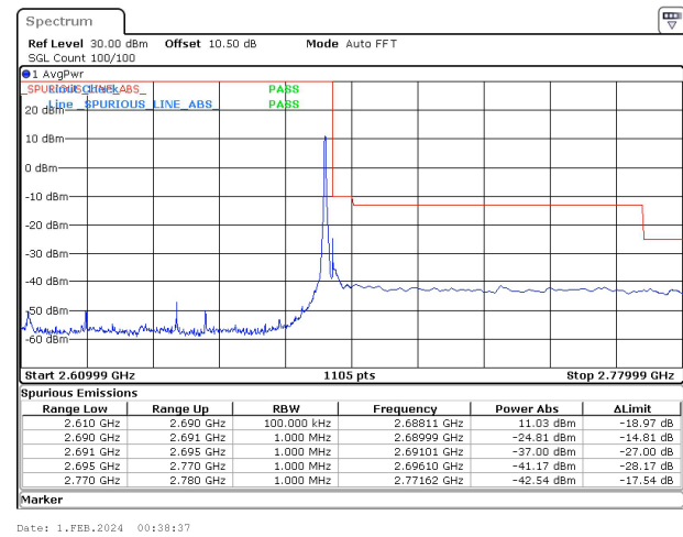
80MHz_30kHz_2649.99MHz_DFT-s-OFDM QPSK_RB1@216~-24.81 dBm
