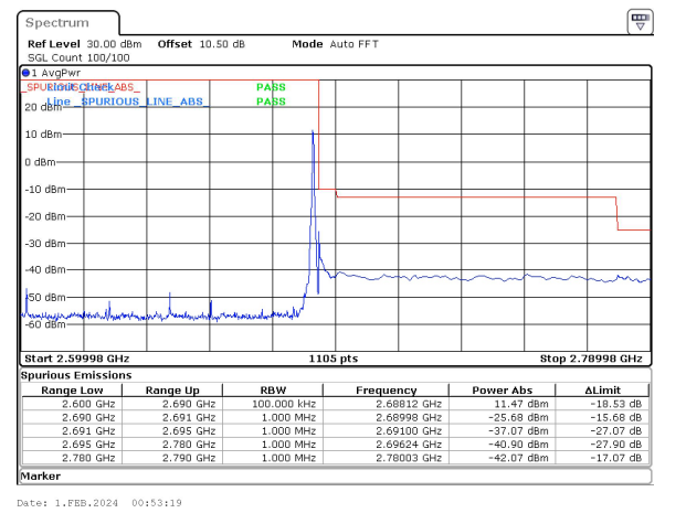
90MHz_30kHz_2644.98MHz_DFT-s-OFDM QPSK_RB1@244~-25.68 dBm
