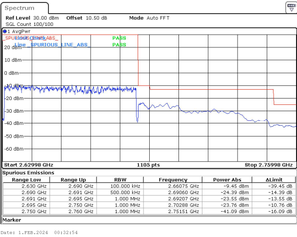
60MHz_30kHz_2659.98MHz_DFT-s-OFDM QPSK_RB162@0&-23.76 dBm
