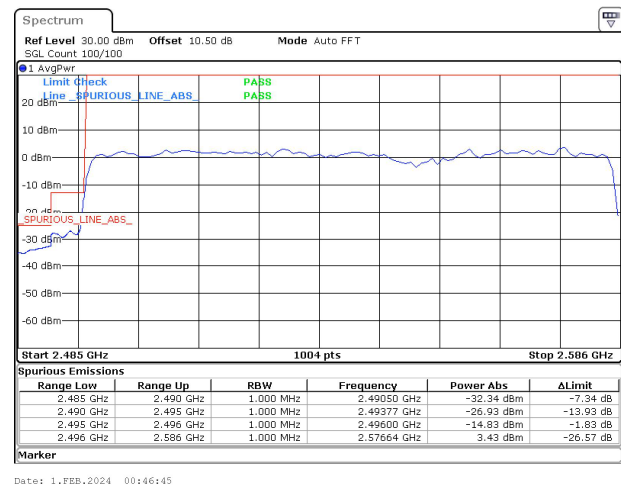
90MHz_30kHz_2541MHz_DFT-s-OFDM QPSK_RB243@0~-14.83 dBm
