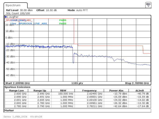
90MHz_30kHz_2644.98MHz_DFT-s-OFDM QPSK_RB243@0~-26.32 dBm
