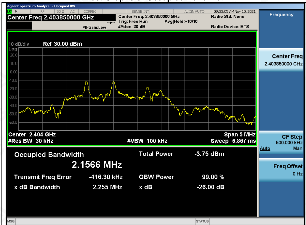
Test_Graph_ANT1_2403.85_OBW
