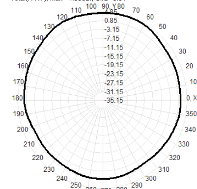
5250.0MHz Total(E2-YZ), Max= 4.26dBi
