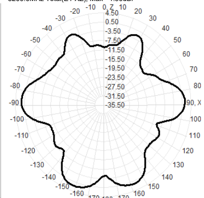
5200.0MHz Total(E1-XZ), Max= 1.90dBi
