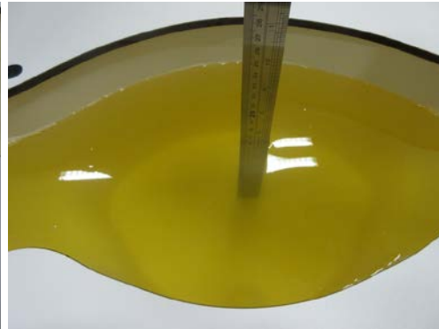
Body 1900MHz~2700MHz_15.3cm
