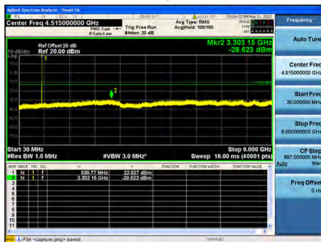
B5 / 10MHz / High CH / 16QAM
