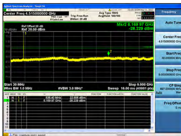
B5 / 1.4MHz / Mid CH / 16QAM
