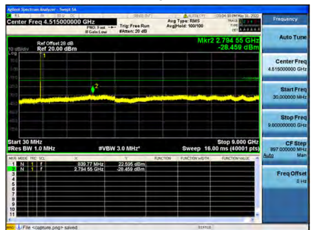
B5 / 10MHz / High CH / 64QAM
