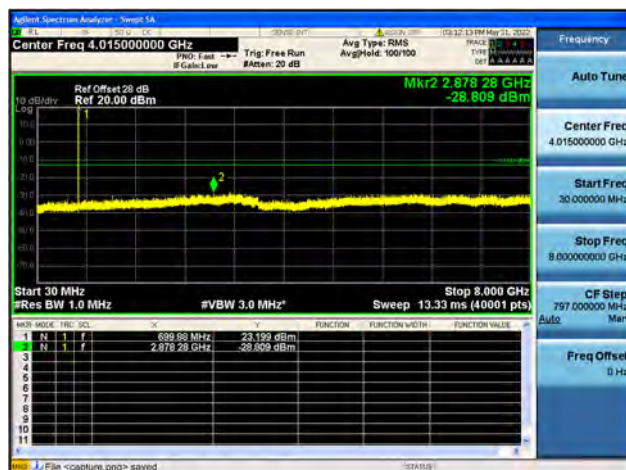
B12 / 10MHz / Low CH / 16QAM
