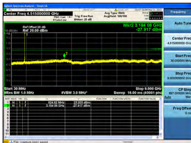
B5 / 3MHz / Low CH / 16QAM
