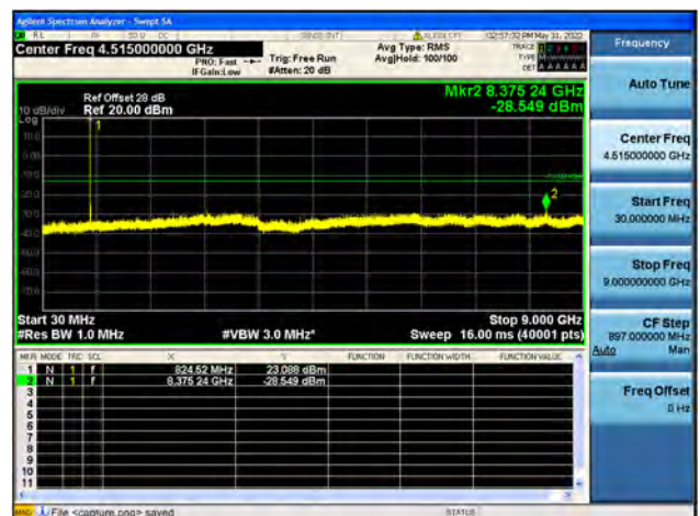
B5 / 3MHz / Low CH / 64QAM
