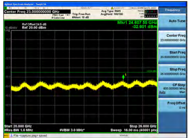
B7-20G-26G / 20MHz / Mid CH / 64QAM
