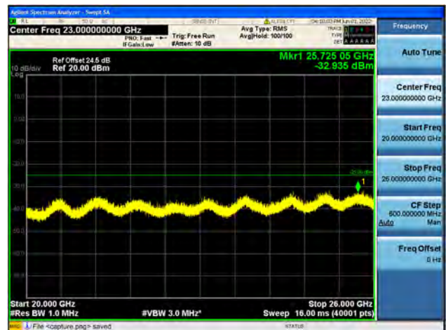
B7-20G-26G / 20MHz / Low CH / 64QAM
