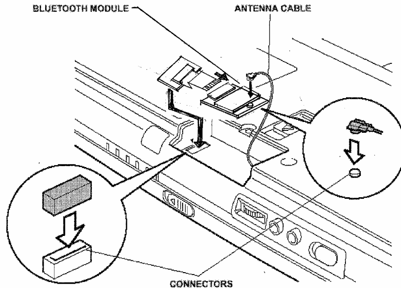
Installing the Bluetooth module (Tecra 9000)
