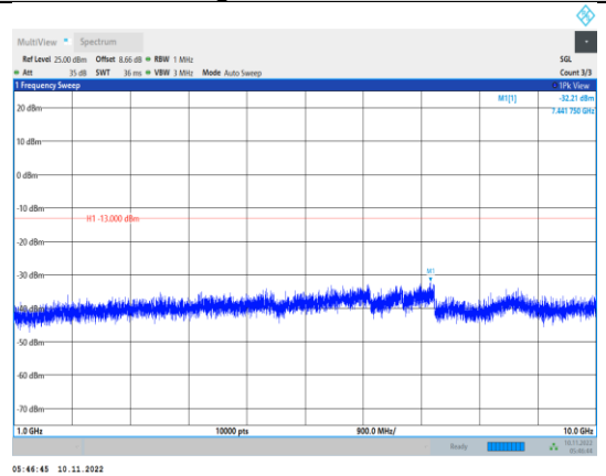
Band26-5MHz-QPSK-26765-1RB#0- Range2:1000~10000MHz
