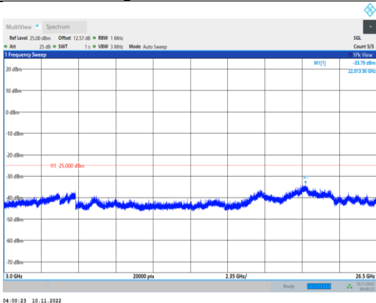
Band38-5MHz-QPSK-38225-1RB#0- Range3:3000~26500MHz
