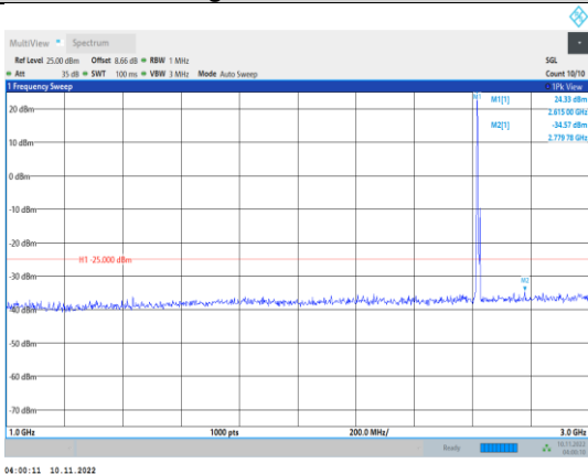
Band38-5MHz-QPSK-38225-1RB#0- Range2:1000~3000MHz
