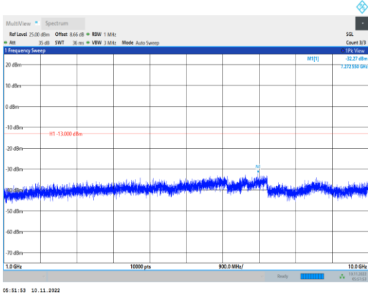
Band26-1.4MHz-QPSK-26697-1RB#0- Range2:1000~10000MHz
