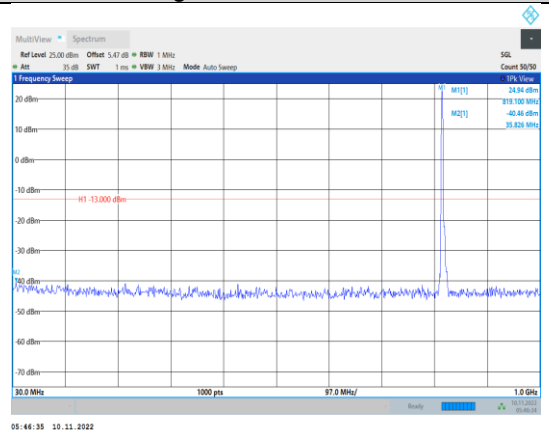
Band26-5MHz-QPSK-26765-1RB#0- Range1:30~1000MHz
