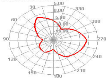
5150.000MHz E1
