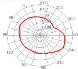
2400.000MHz E1
