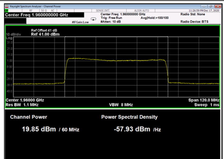
Figure 202: 256QAM 60MHz B.W.; 1960.0MHz, 60kHz
