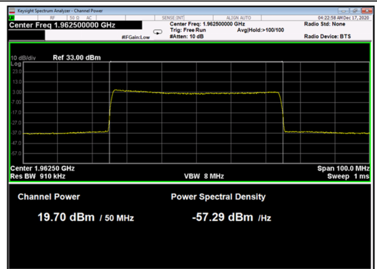
Figure 262: QPSK 50MHz B.W.; 1962.5MHz, 30kHz
