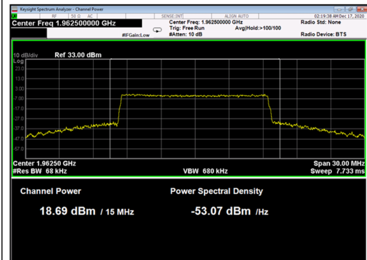
Figure 227: QPSK 15MHz B.W.; 1962.5MHz, 60kHz
