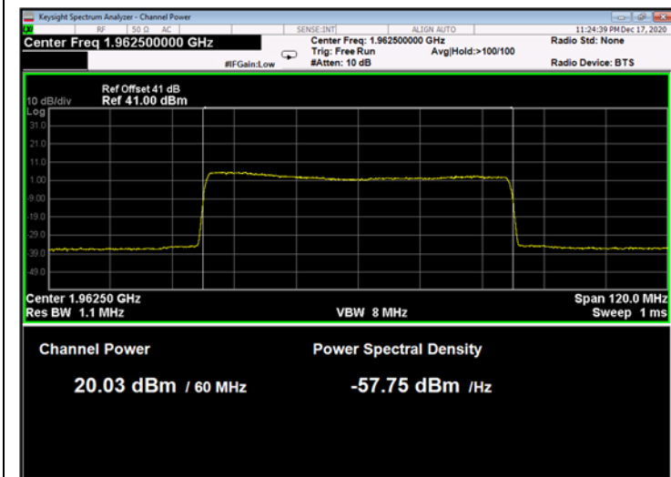
Figure 203: 256QAM 60MHz B.W.; 1962.5MHz, 30kHz
