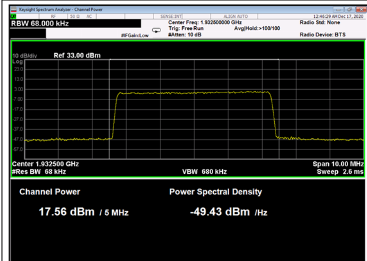
Figure 207: QPSK 5MHz B.W.; 1932.5MHz, 15kHz
