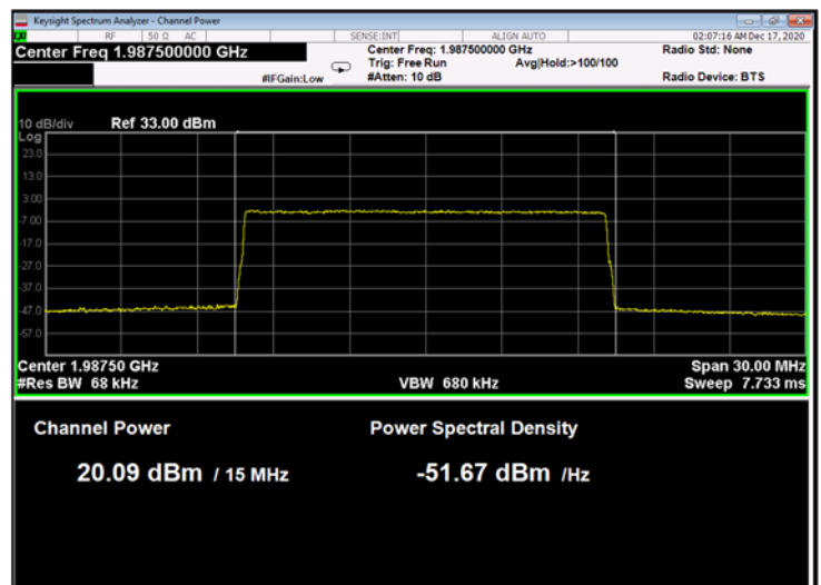
Figure 228: QPSK 15MHz B.W.; 1987.5MHz, 15kHz
