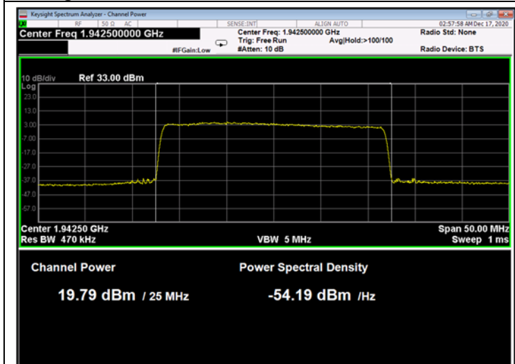
Figure 241: QPSK 25MHz B.W.; 1942.5MHz, 30kHz
