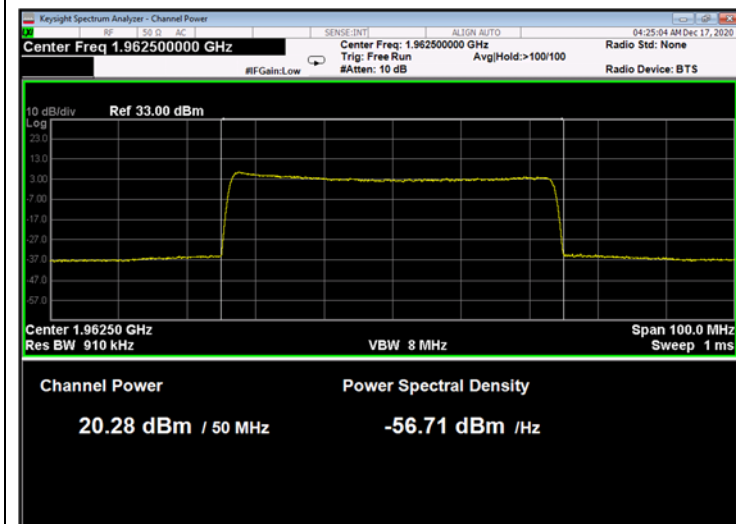
Figure 263: QPSK 50MHz B.W.; 1962.5MHz, 60kHz
