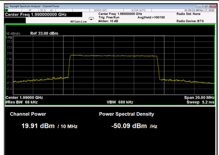
Figure 220: QPSK 10MHz B.W.; 1990.0MHz, 30kHz
