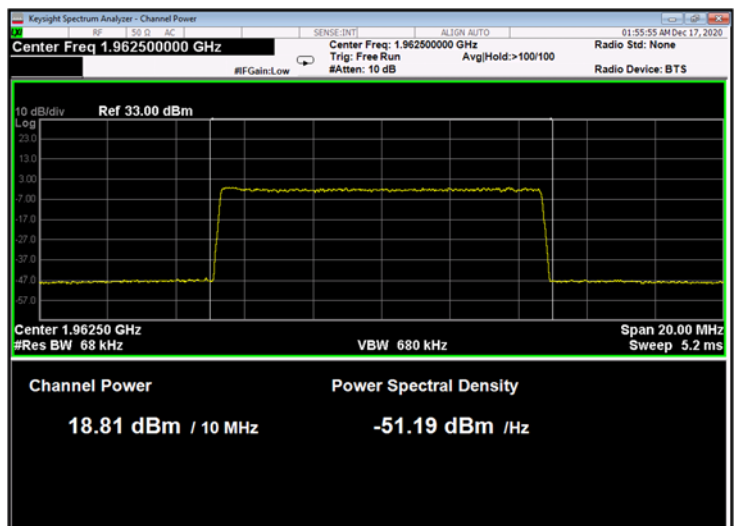
Figure 216: QPSK 10MHz B.W.; 1962.5MHz, 15kHz
