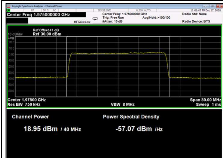
Figure 191: 256QAM 40MHz B.W.; 1975.0MHz, 60kHz
