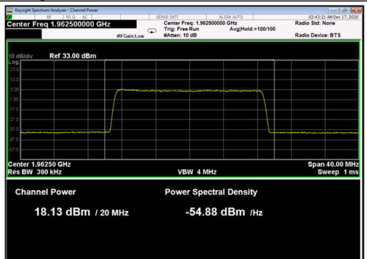
Figure 236: QPSK 20MHz B.W.; 1962.5MHz, 60kHz
