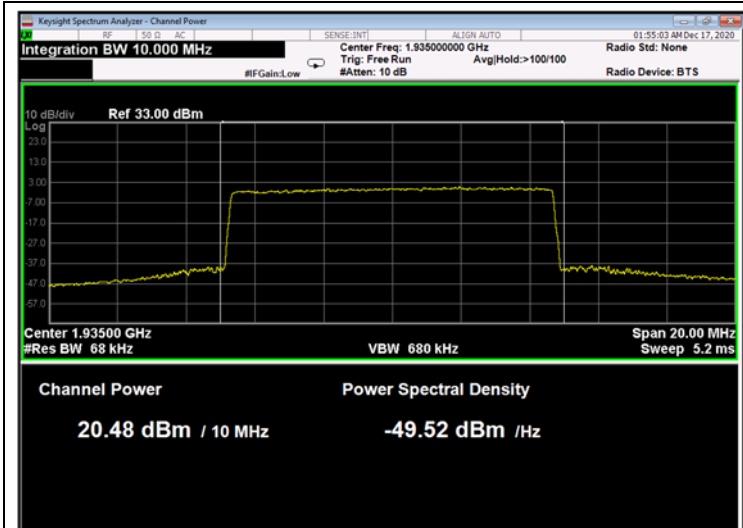
Figure 213: QPSK 10MHz B.W.; 1935.0MHz, 15kHz
