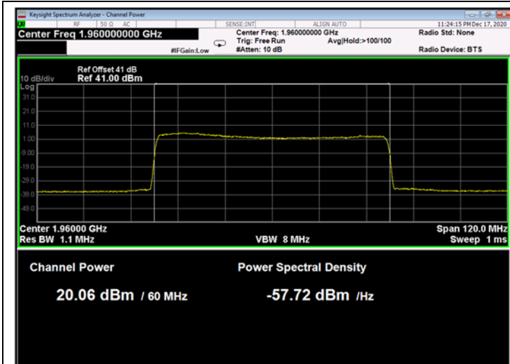
Figure 201: 256QAM 60MHz B.W.; 1960.0MHz, 30kHz
