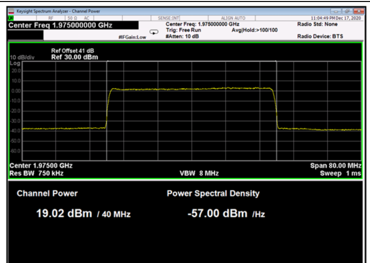
Figure 190: 256QAM 40MHz B.W.; 1975.0MHz, 30kHz
