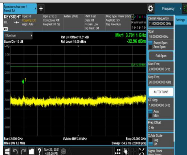
Band25-1.4MHz-QPSK-26047-6RB#0-Range3:2000~20000MHz
