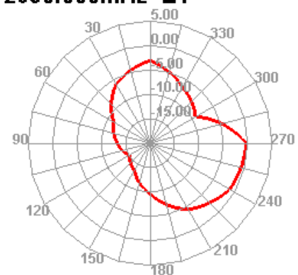
2690.000MHz E1
