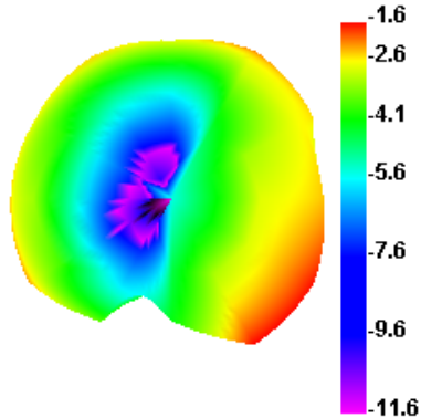
820.000MHz E1
