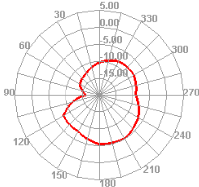
960.000MHz E2
