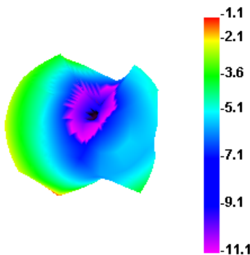
960.000MHz E1
