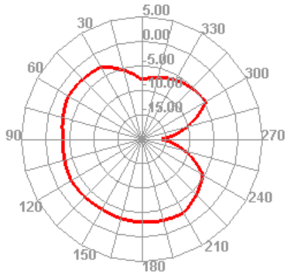
820.000MHz H
