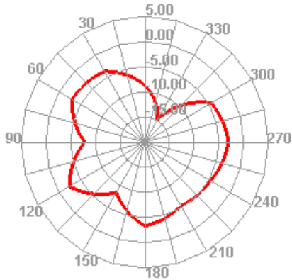
820.000MHz E1
