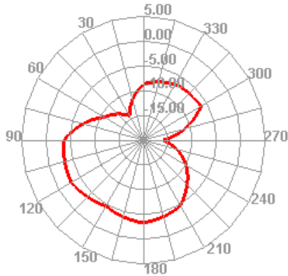
820.000MHz E2
