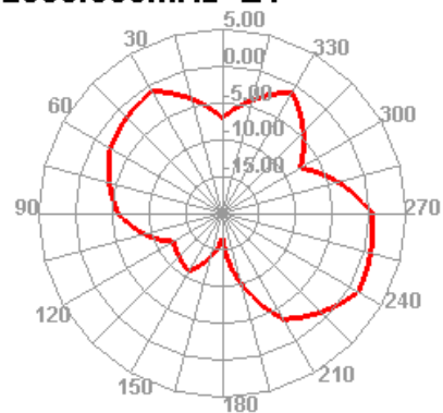
2300.000MHz E1
