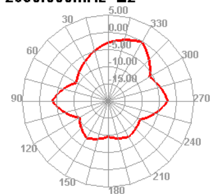
2690.000MHz E2
