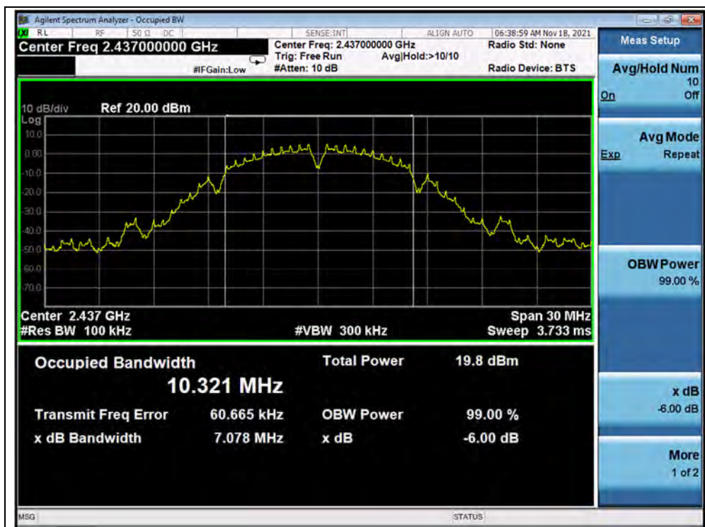
(Channel 6, 802.11b)
