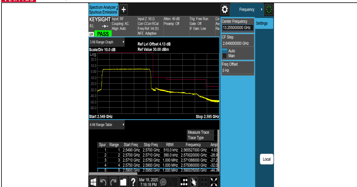
Band7-20MHz-QPSK-21350-1RB#99-PASS
