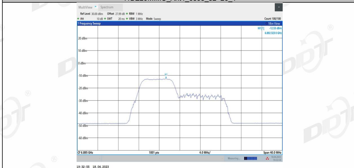
11BE20MIMO Ant4 6895 52+26 2
