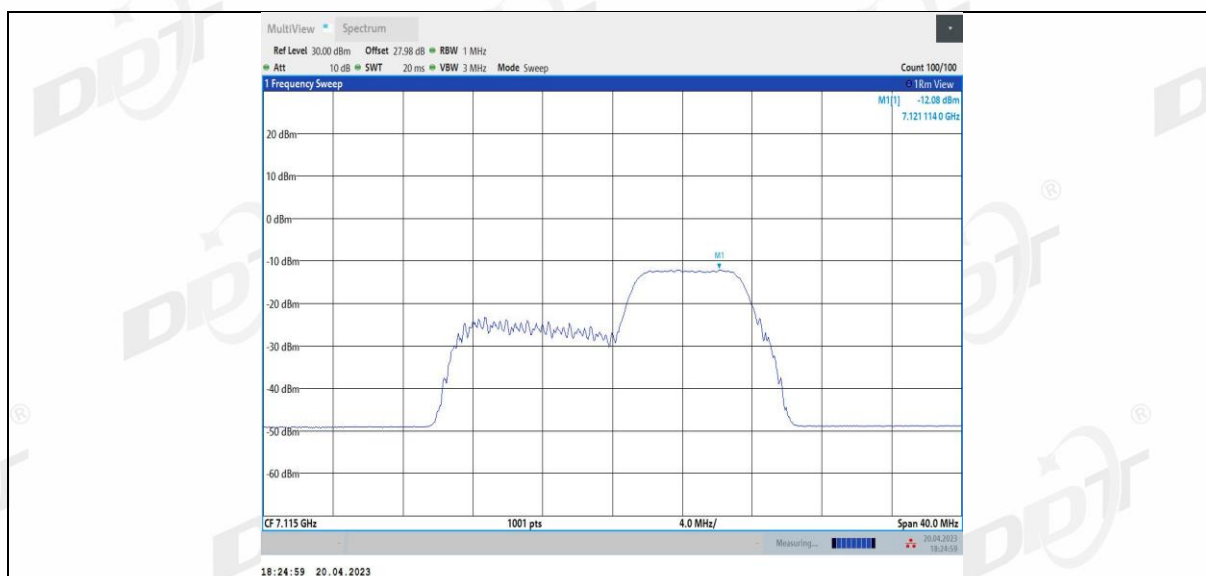
11BE20MIMO Ant3 7115 106+26 1
