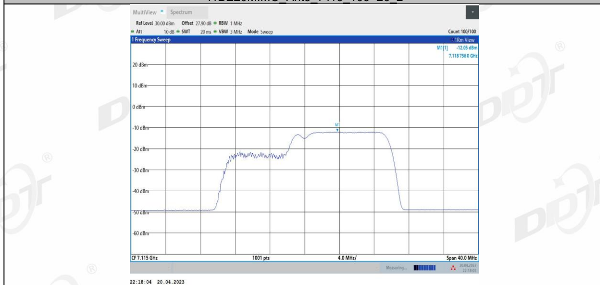
11BE20MIMO Ant4 7115 52+26 1
