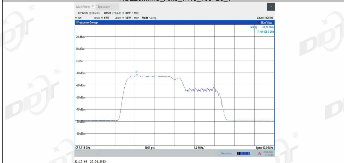
11BE20MIMO Ant3 7115 106+26 2
