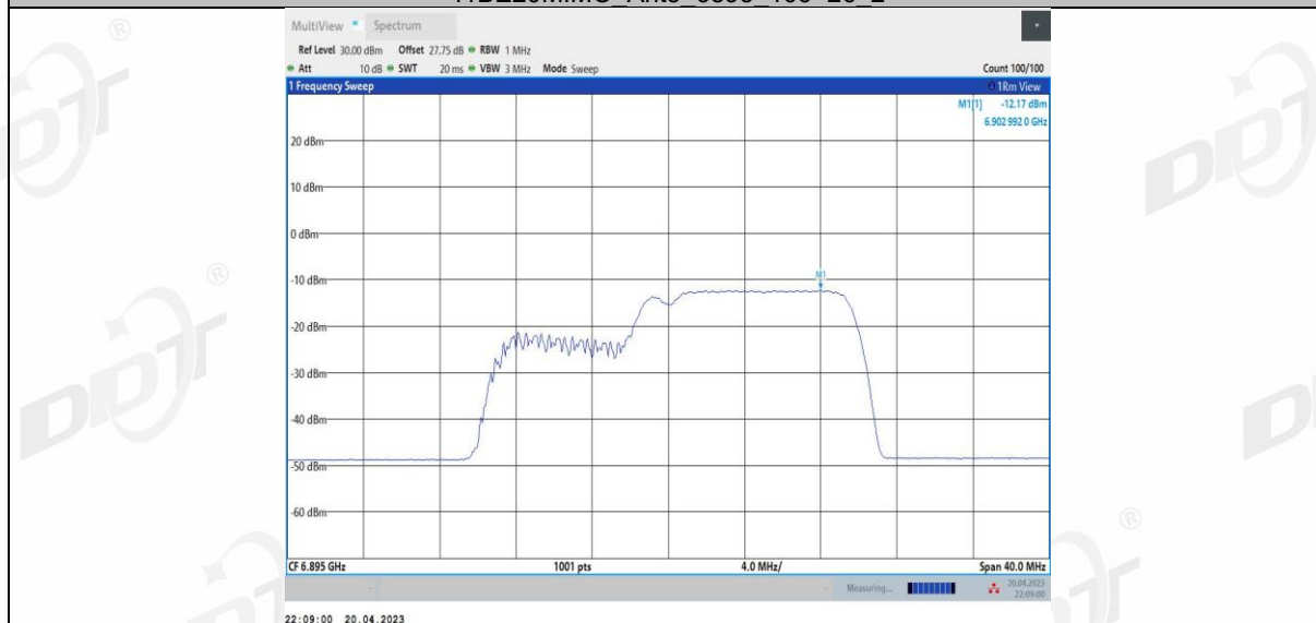
11BE20MIMO Ant4 6895 52+26 1
