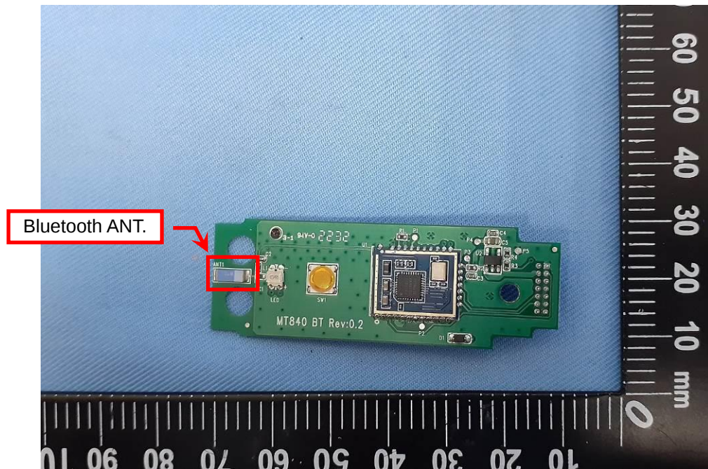
EUT Photo (20)
