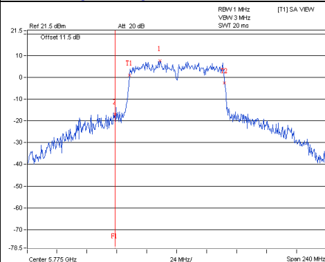
802.11ac(VHT80)_Chain2 / CH155
