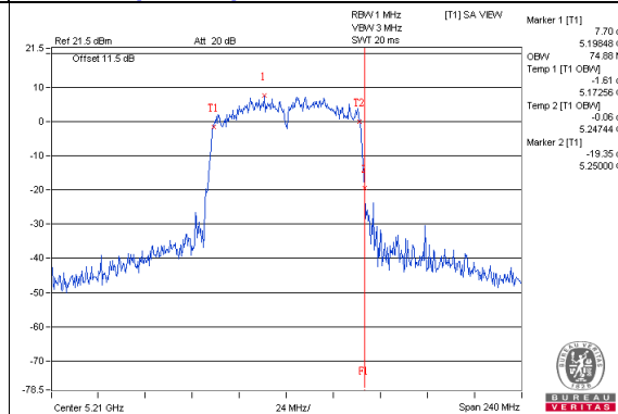
802.11ac(VHT80)_Chain3 / CH42
