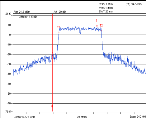
802.11ac(VHT80)_Chain3 / CH155
