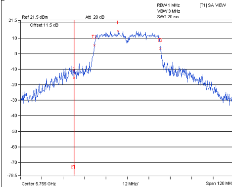
802.11ac(VHT40)_Chain3 / CH151
