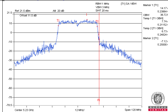
802.11ac(VHT40)_Chain3 / CH46
