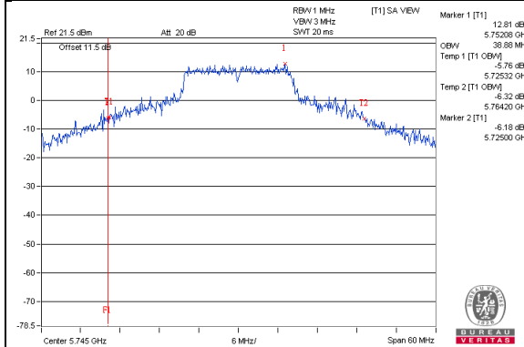
802.11a_Chain2 / CH149
