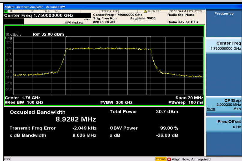
Band4-10MHz-QPSK-20350-50RB#0-8.9282
