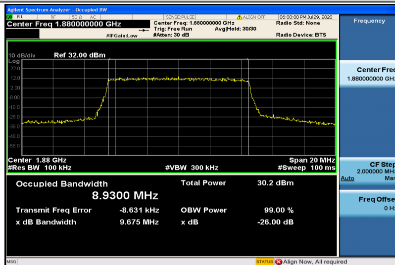
Band2-10MHz-QPSK-18900-50RB#0-8.9300
