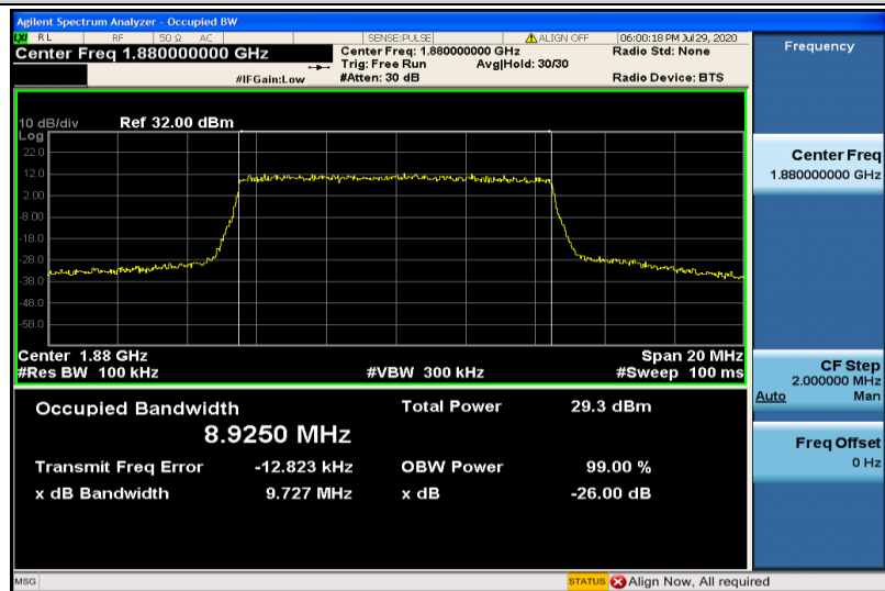
Band2-10MHz-16QAM-18900-50RB#0-8.9250
