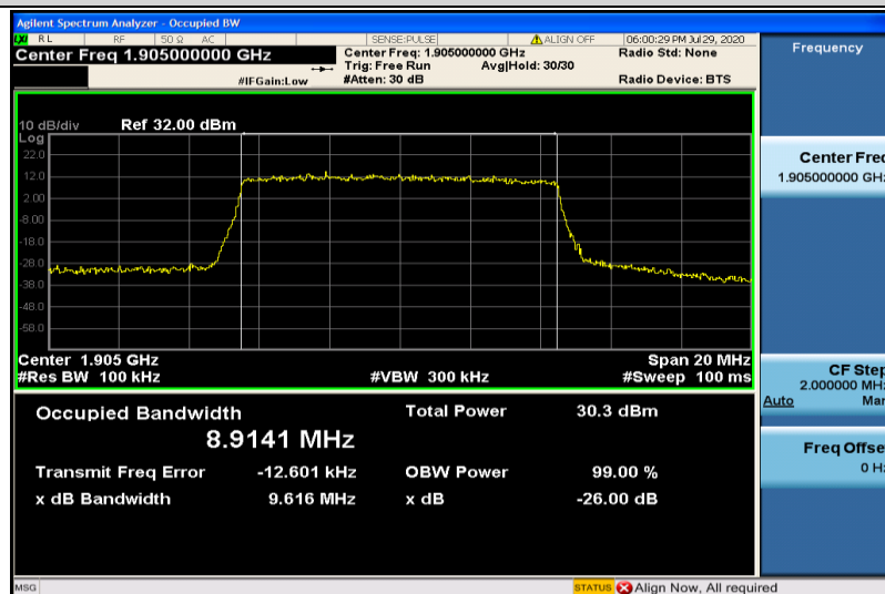
Band2-10MHz-QPSK-19150-50RB#0-8.9141
