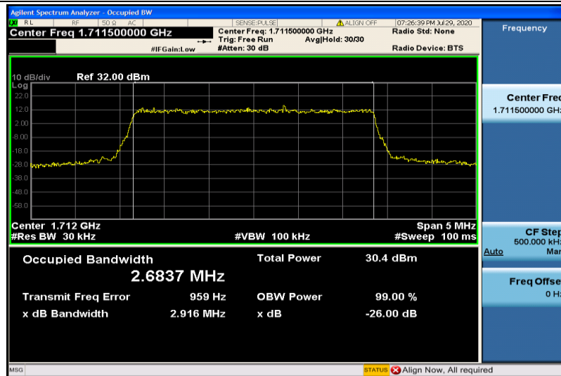
Band4-3MHz-QPSK-19965-15RB#0-2.6837
