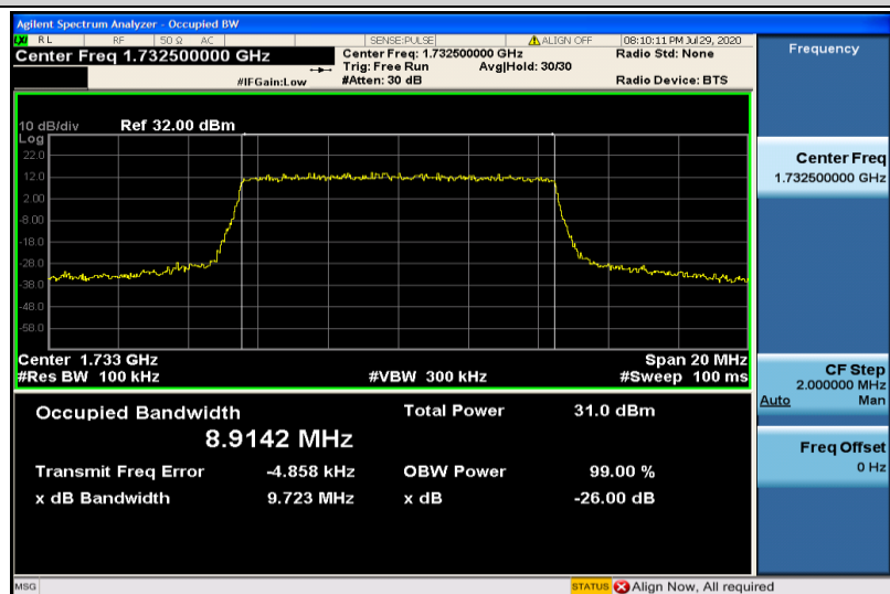
Band4-10MHz-QPSK-20175-50RB#0-8.9142
