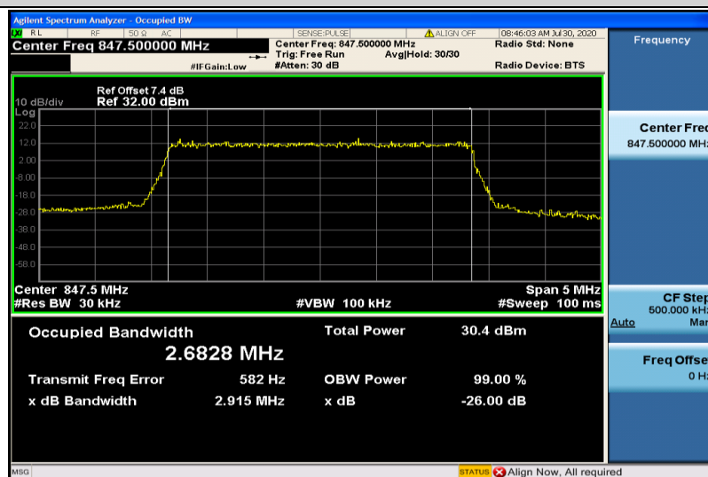
Band5-3MHz-QPSK-20635-15RB#0-2.6828
