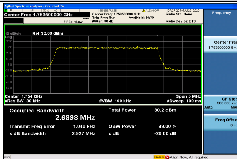
Band4-3MHz-QPSK-20385-15RB#0-2.6898
