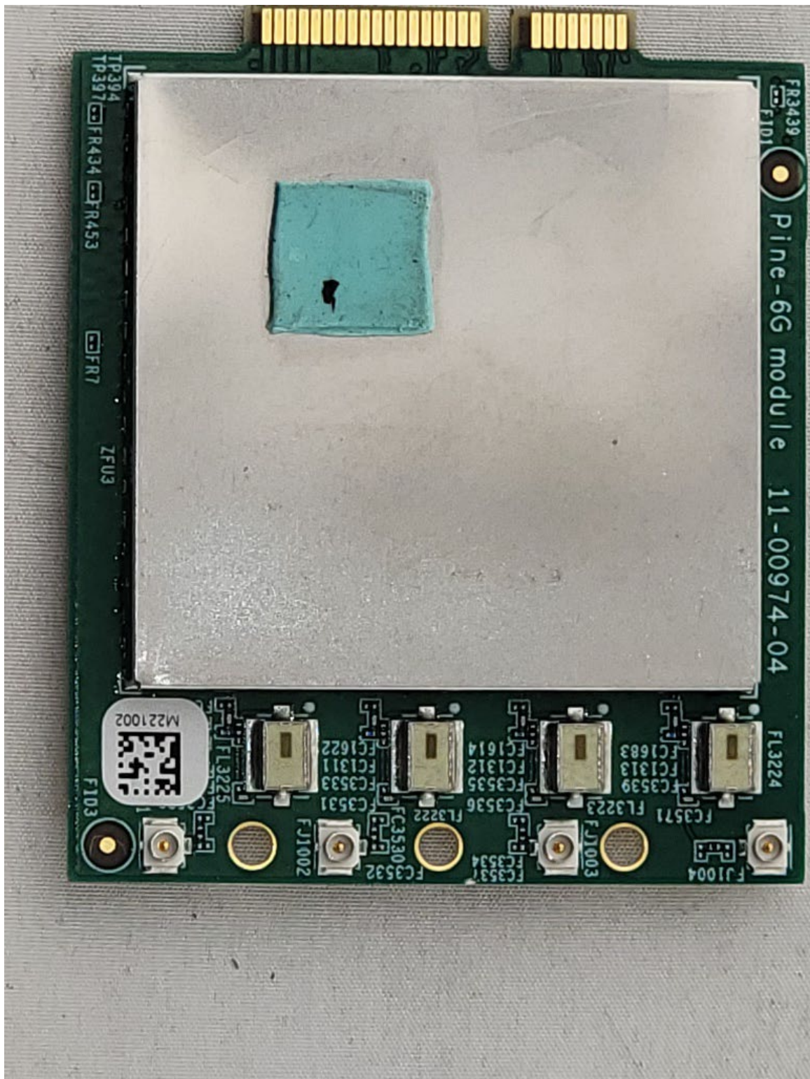
6G PCB Top EMI can(s) installed
