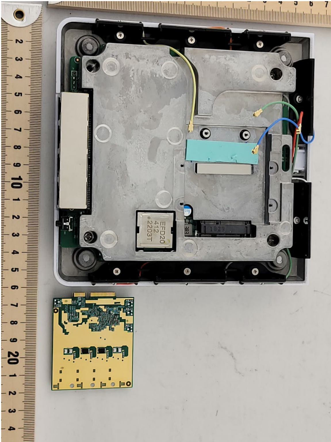
6G Module removed
