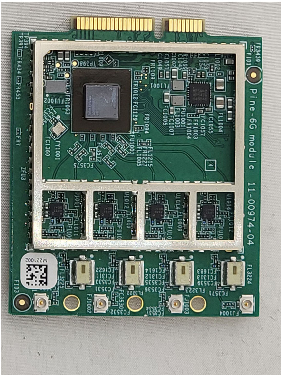
6G PCB Top EMI can(s) removed
