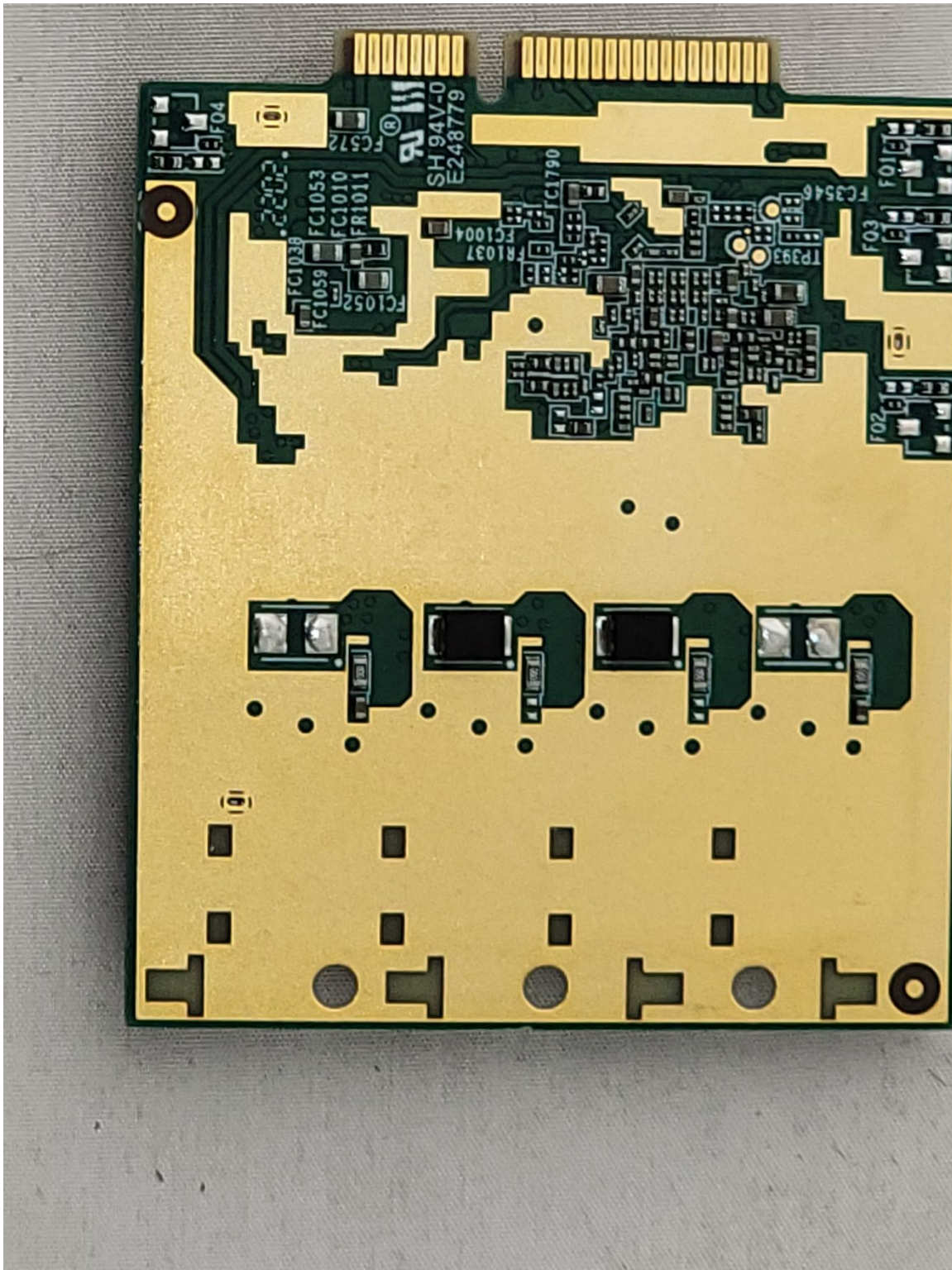
6G PCB Bottom
