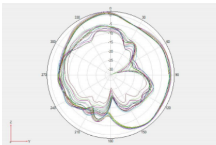
Phi 90 2D 图
