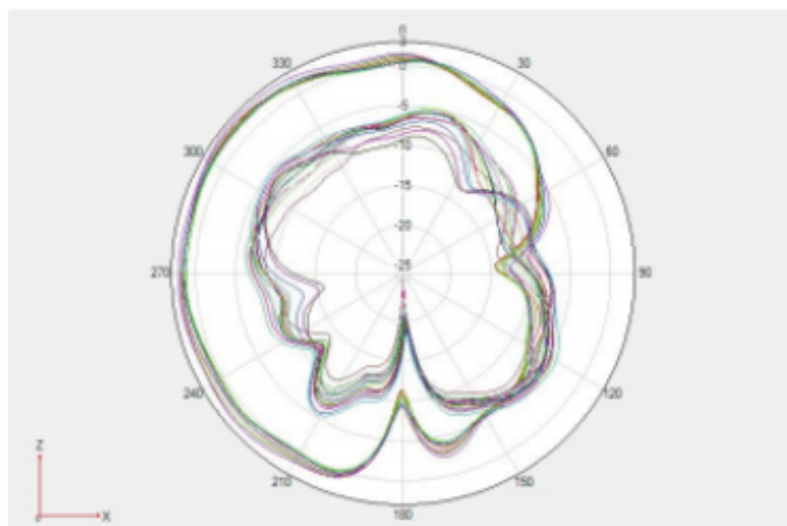
Phi 0 2D 图
