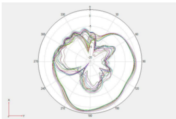
Theta 90 2D 图
