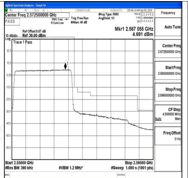
Band7_20MHz_16QAM_21350_100RB#0
