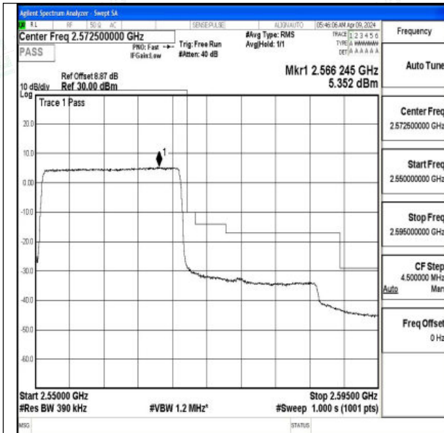
Band7_20MHz_QPSK_21350_100RB#0
