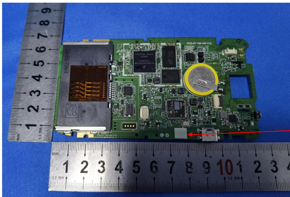
BT/WIFI antenna
