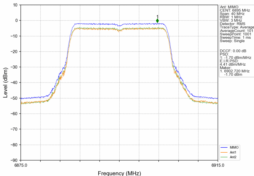
802.11be(EHT20)_LCH_6895MHz_RU242_Left_MIMO_NTNV
