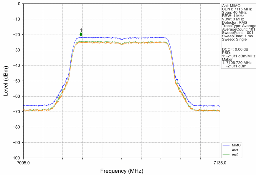
802.11be(EHT20)_HCH_7115MHz_RU242_Left_MIMO_NTNV
