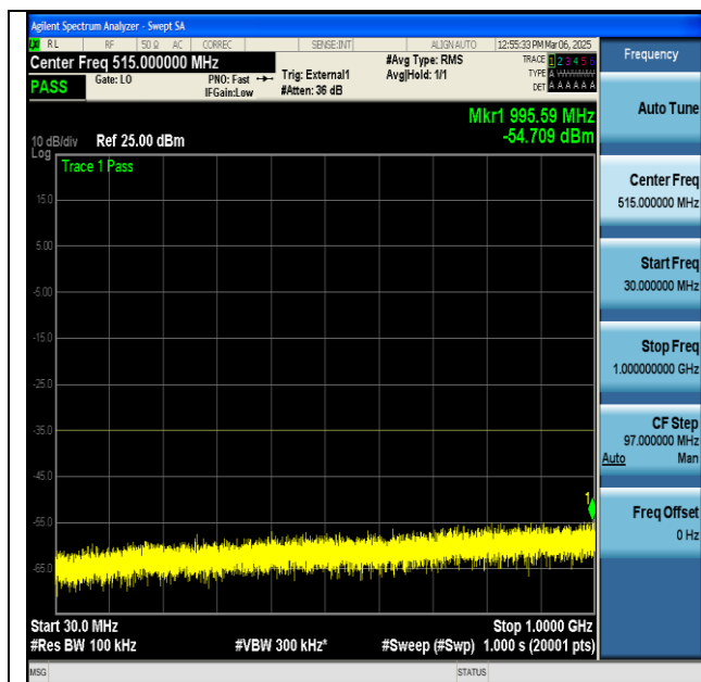
NTNV-n41-PC2-30-100-M-CP-QPSK-Edge_1RB_Left-30-1000-PASS
