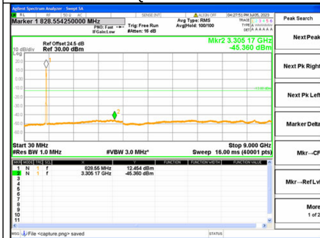
5B / 10+10MHz / QPSK / Low CH / 50#0-50#0
