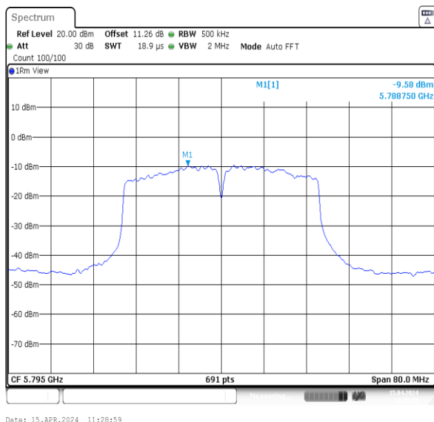
11N40MIMO-Ant1-5795-PASS
