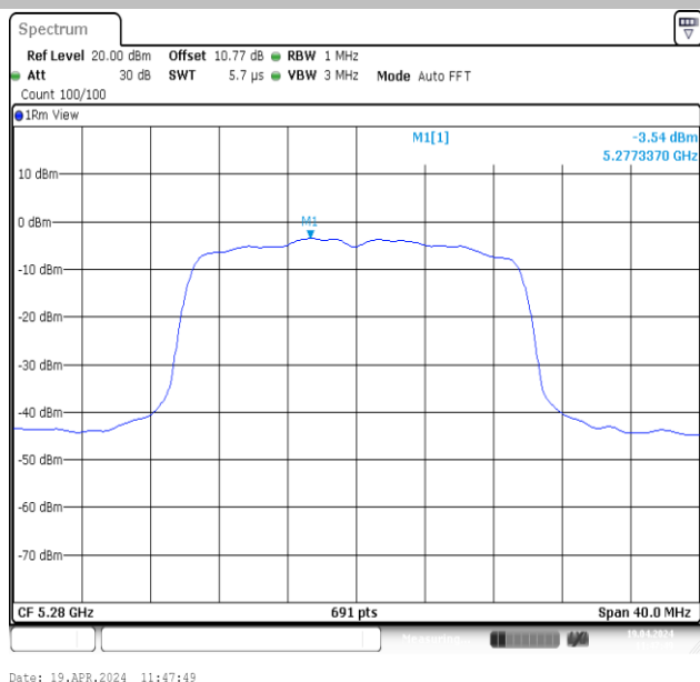
11AX20MIMO-Ant1-5280-PASS
