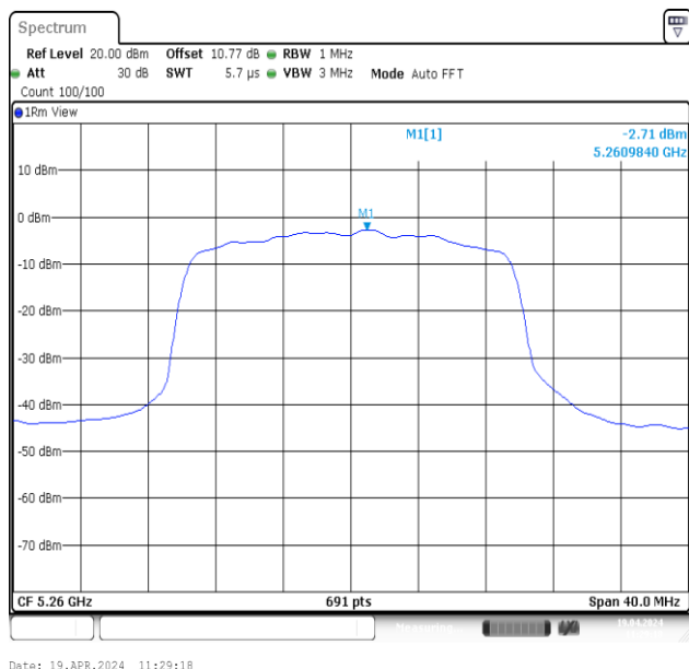
11AX20MIMO-Ant1-5260-PASS
