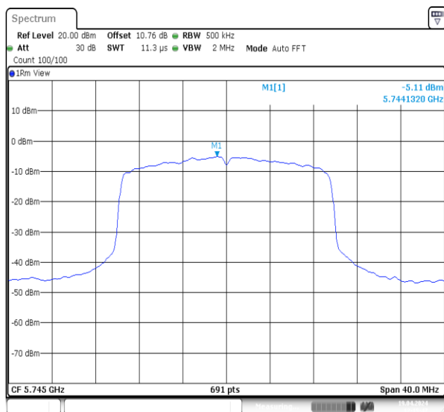
11AX20MIMO-Ant1-5745-PASS
