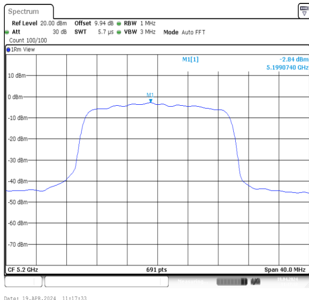
11AX20MIMO-Ant1-5200-PASS
