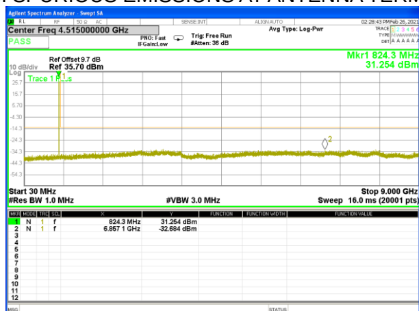
GSM850_Low
