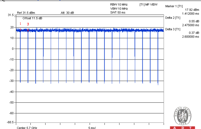
802.11ac (VHT20)
