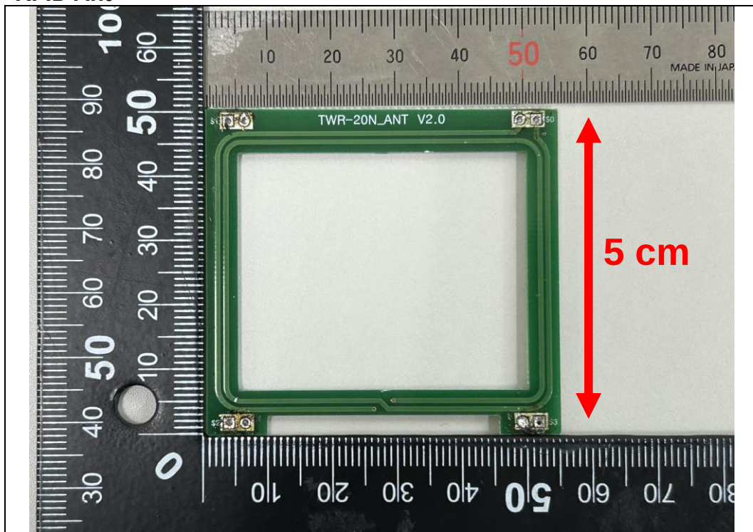
RFID Ant
