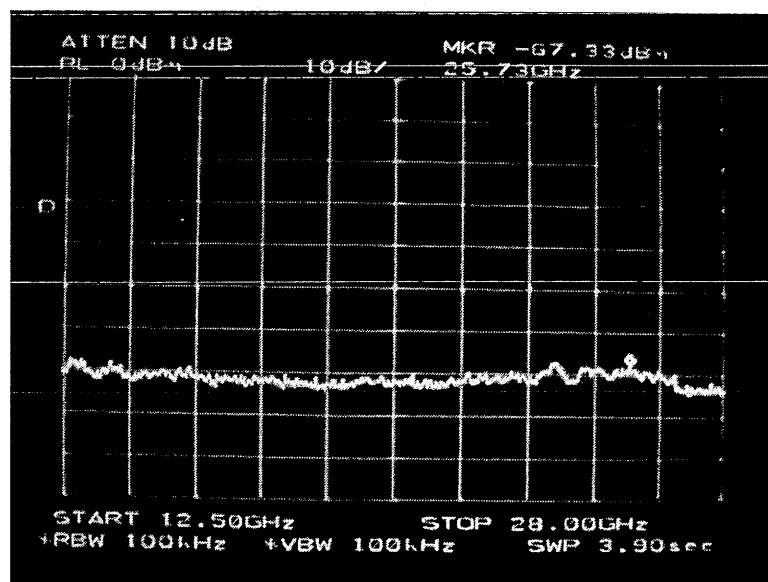
0.07 μS Pulse
