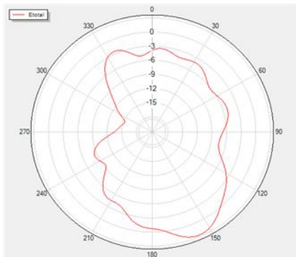
Theta=90 Freq=2400MHz
