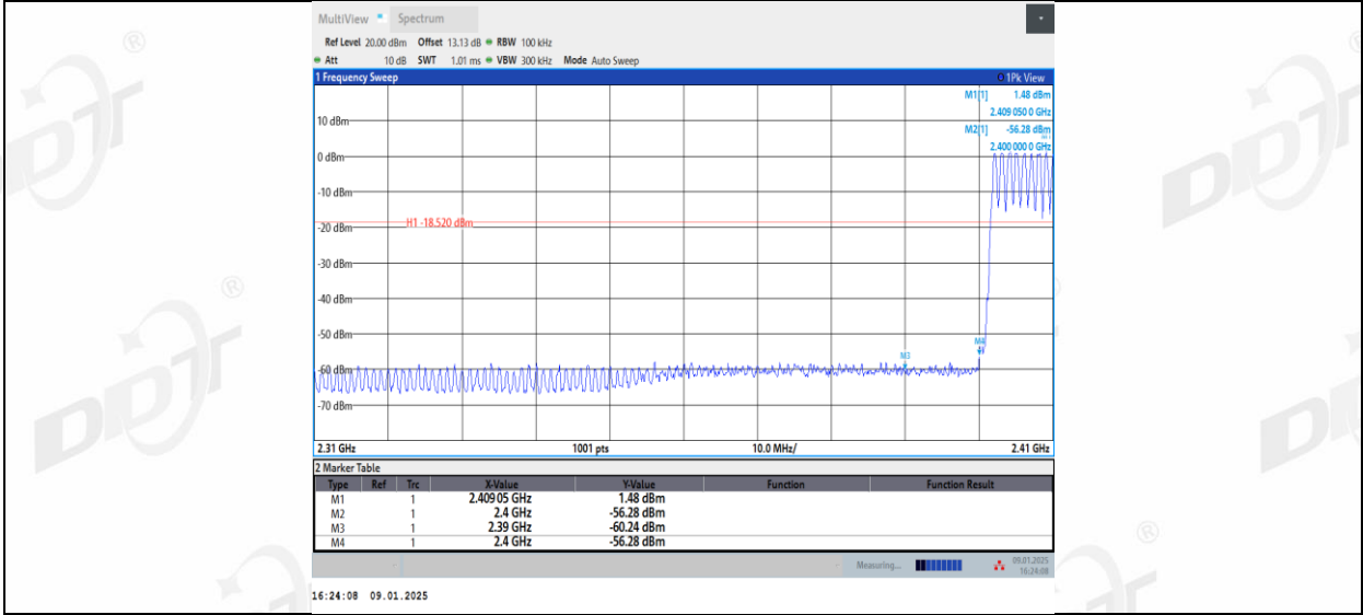
DH5_Right side_Low_Hop_2402
