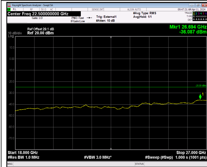
Band41_20MHz_16QAM_41490_1RB#0_18000~27000_18000~27000
