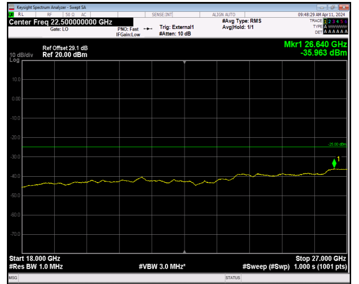
Band41_20MHz_64QAM_41490_1RB#0_18000~27000_18000~27000
