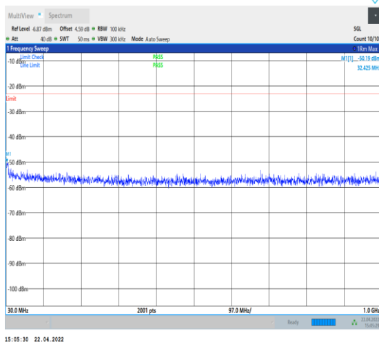
1-N25--15-40-L-1-DFT-PI2BPSK-Inner_1RB_Left-1 @1-30-1000-Ant0--50.19--23-PASS
