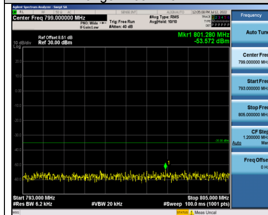
Band13-10MHz-QPSK-23230-1RB#0- Range5:793~805MHz
