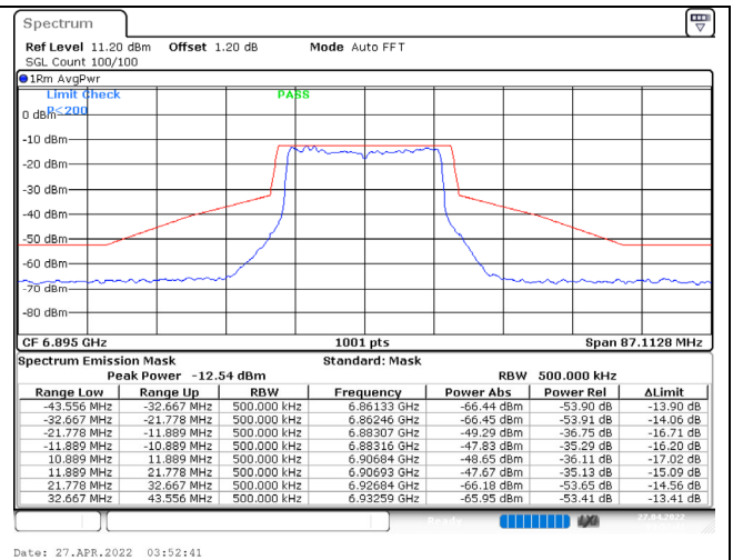
802.11ax (20MHz) / 6895MHz / Chain B / NSS-1
