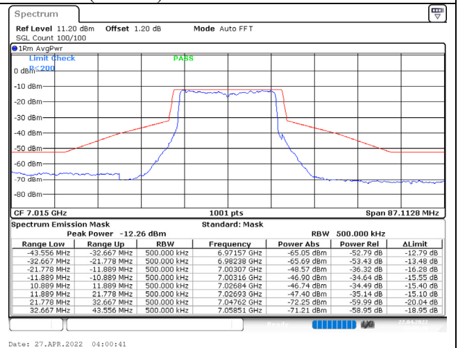
802.11ax (20MHz) / 7015MHz / Chain B / NSS-1
