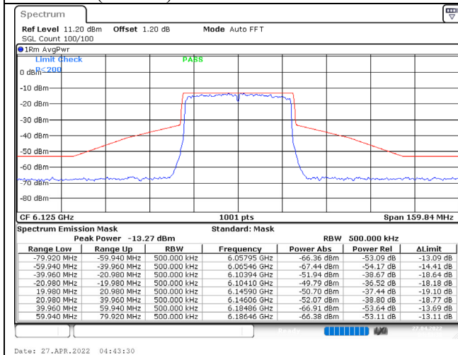
802.11ax (40MHz) / 6125MHz / Chain A / NSS-1
