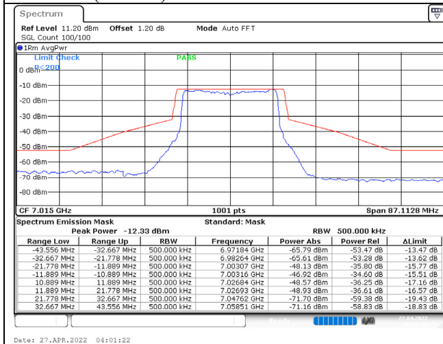
802.11ax (20MHz) / 7015MHz / Chain A / NSS-1
