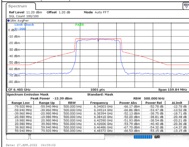
802.11ax (40MHz) / 6405MHz / Chain C / NSS-1
