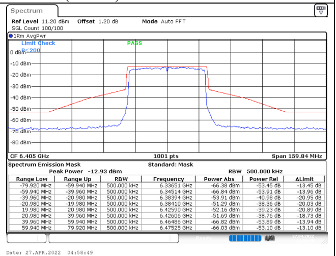
802.11ax (40MHz) / 6405MHz / Chain D / NSS-1
