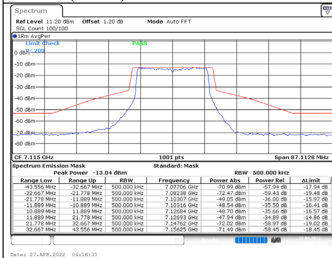
802.11ax (20MHz) / 7115MHz / Chain C / NSS-1
