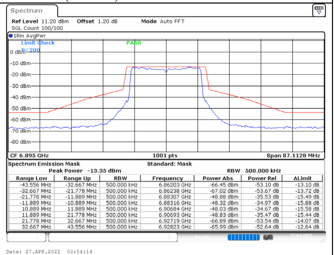
802.11ax (20MHz) / 6895MHz / Chain D / NSS-1
