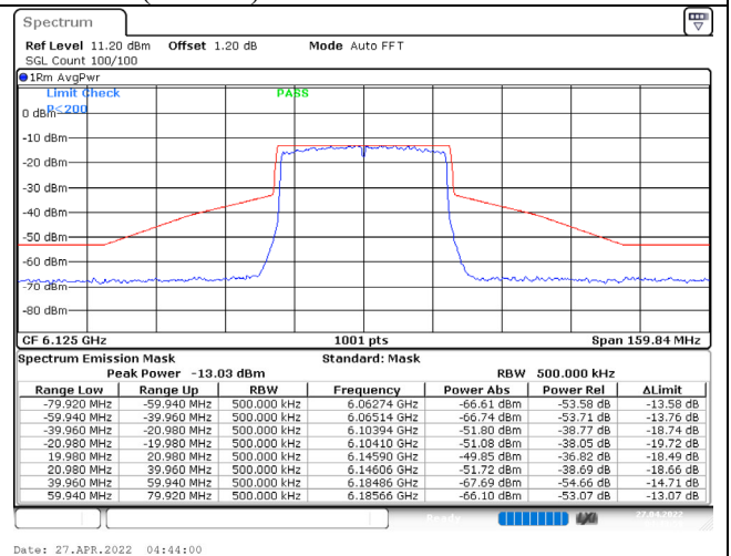
802.11ax (40MHz) / 6125MHz / Chain B / NSS-1
