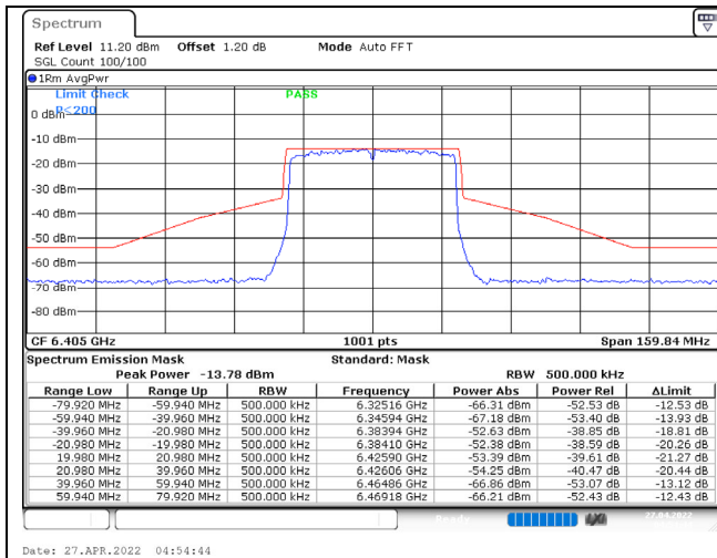
802.11ax (40MHz) / 6405MHz / Chain A / NSS-1
