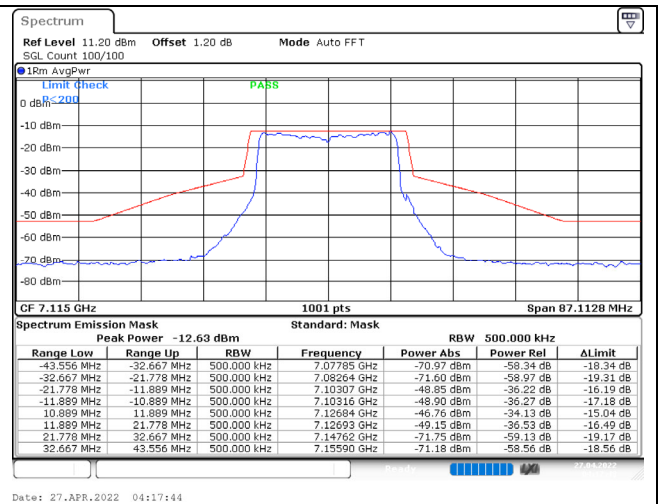
802.11ax (20MHz) / 7115MHz / Chain B / NSS-1
