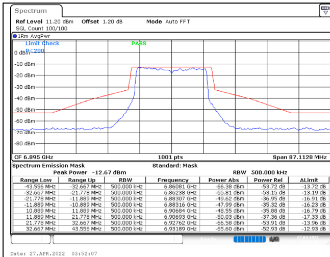
802.11ax (20MHz) / 6895MHz / Chain A / NSS-1
