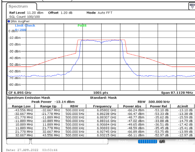
802.11ax (20MHz) / 6895MHz / Chain C / NSS-1
