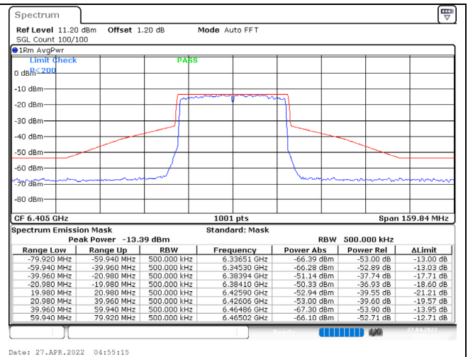
802.11ax (40MHz) / 6405MHz / Chain B / NSS-1
