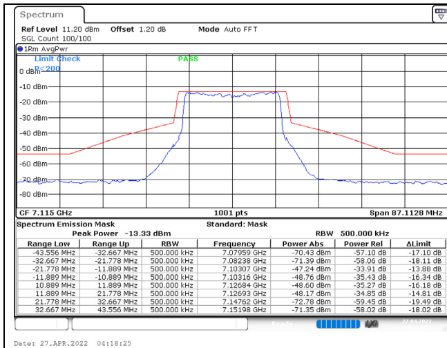
802.11ax (20MHz) / 7115MHz / Chain A / NSS-1
