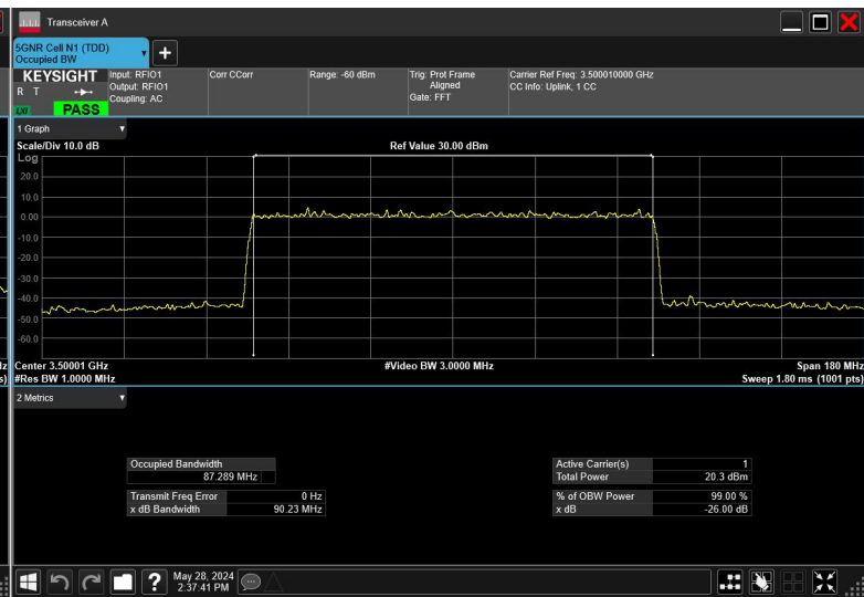
90MHz_30kHz_3500MHz_CP-OFDM QPSK_RB245@0
