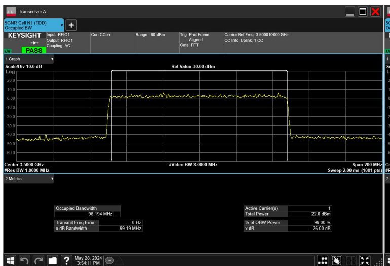
100MHz_30kHz_3500MHz_DFT-s-OFDM QPSK_RB270@0
