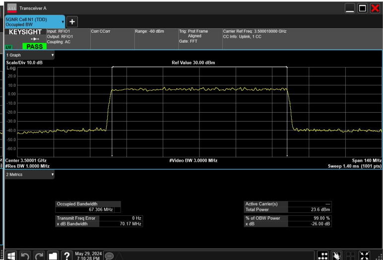
70MHz_30kHz_3500MHz_CP-OFDM QPSK_RB189@0
