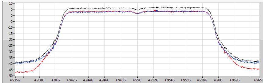
4.94-4.99GHz_802.11j_20MHz_Nss1_2TX 4950MHz
