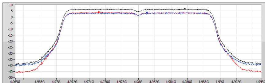
4.94-4.99GHz_802.11j_20MHz_Nss1_2TX 4980MHz
