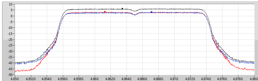
4.94-4.99GHz_802.11j_20MHz_Nss1_2TX 4965MHz
