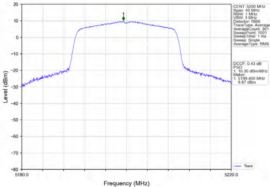
802.11ax(HE20)_MCH_5200MHz_RU242_Left_Ant2_NTNV
