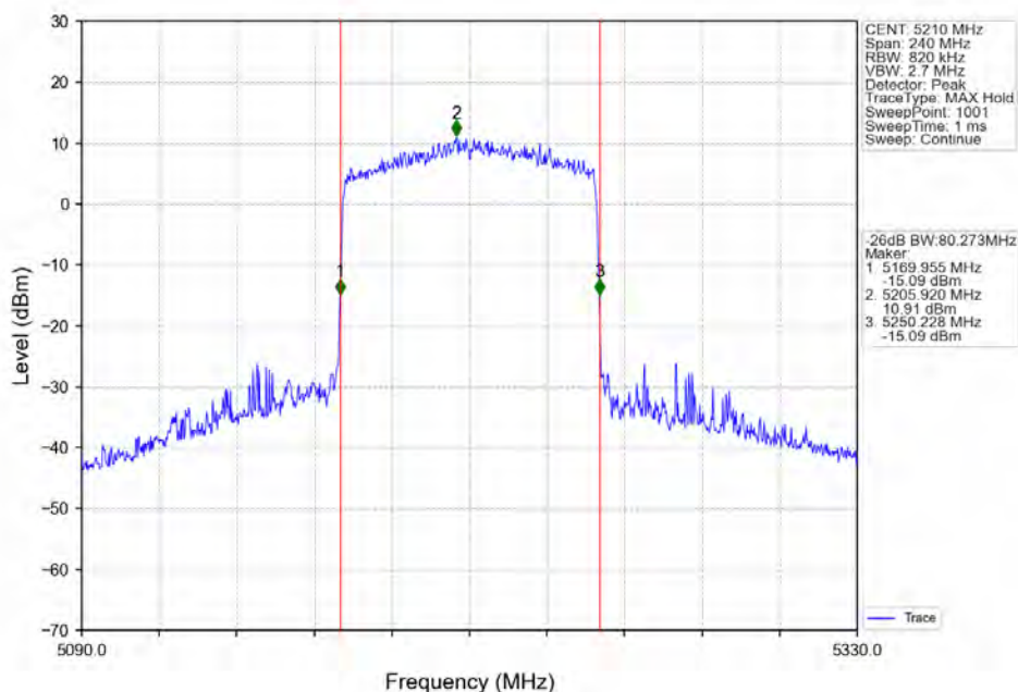
802.11ax(HE80)_MCH_5210MHz_RU996_Left_Ant2_NTNV
