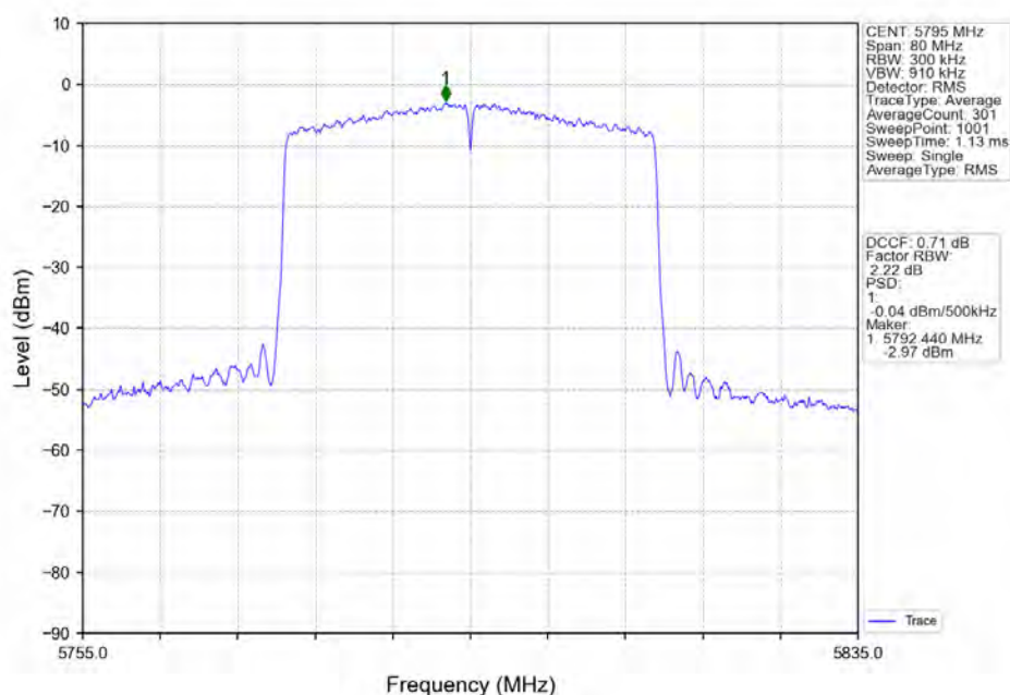
802.11ax(HE40)_HCH_5795MHz_RU484_Left_Ant2_NTNV
