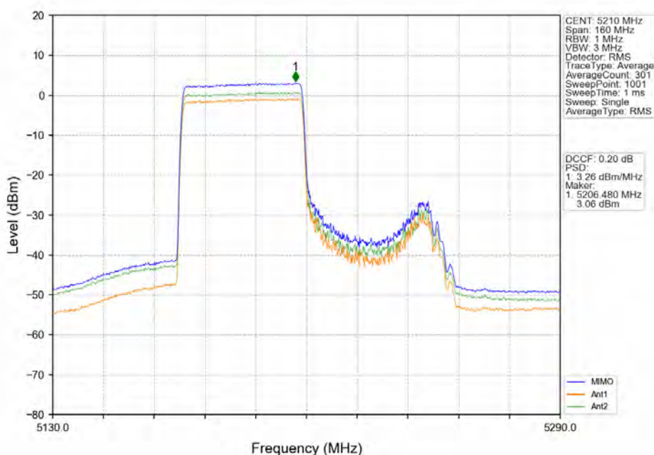
802.11ax(HE80)_MCH_5210MHz_RU484_Left_MIMO_NTNV
