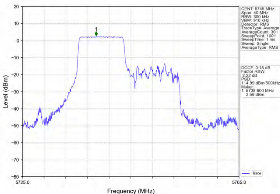
802.11ax(HE20)_LCH_5745MHz_RU106_Left_Ant2_NTNV
