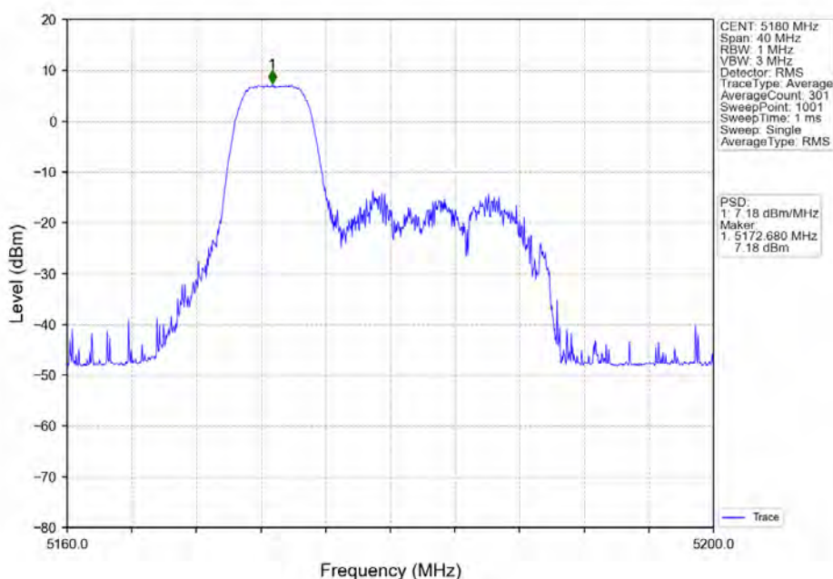
802.11ax(HE20)_LCH_5180MHz_RU52_Left_Ant1_NTNV
