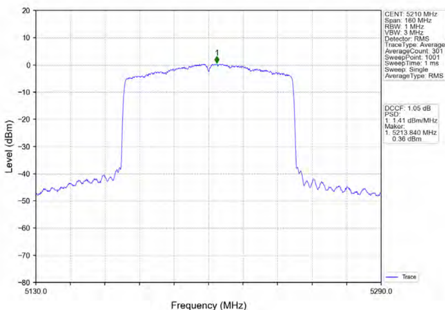
802.11ax(HE80)_MCH_5210MHz_RU996_Left_Ant2_NTNV
