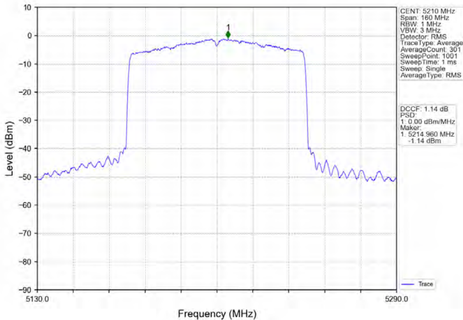
802.11ax(HE80)_MCH_5210MHz_RU996_Left_Ant1_NTNV
