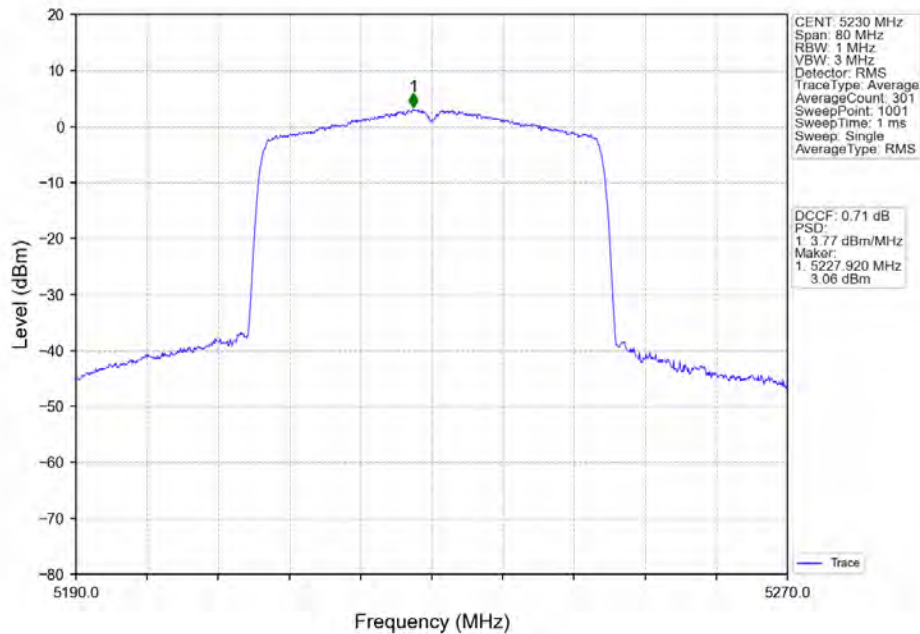
802.11ax(HE40)_HCH_5230MHz_RU484_Left_Ant1_NTNV
