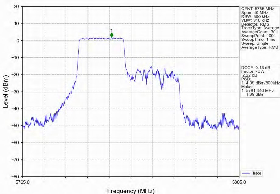
802.11ax(HE20)_MCH_5785MHz_RU106_Left_Ant2_NTNV
