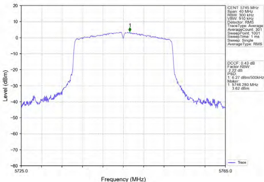
802.11ax(HE20)_LCH_5745MHz_RU242_Left_Ant2_NTNV
