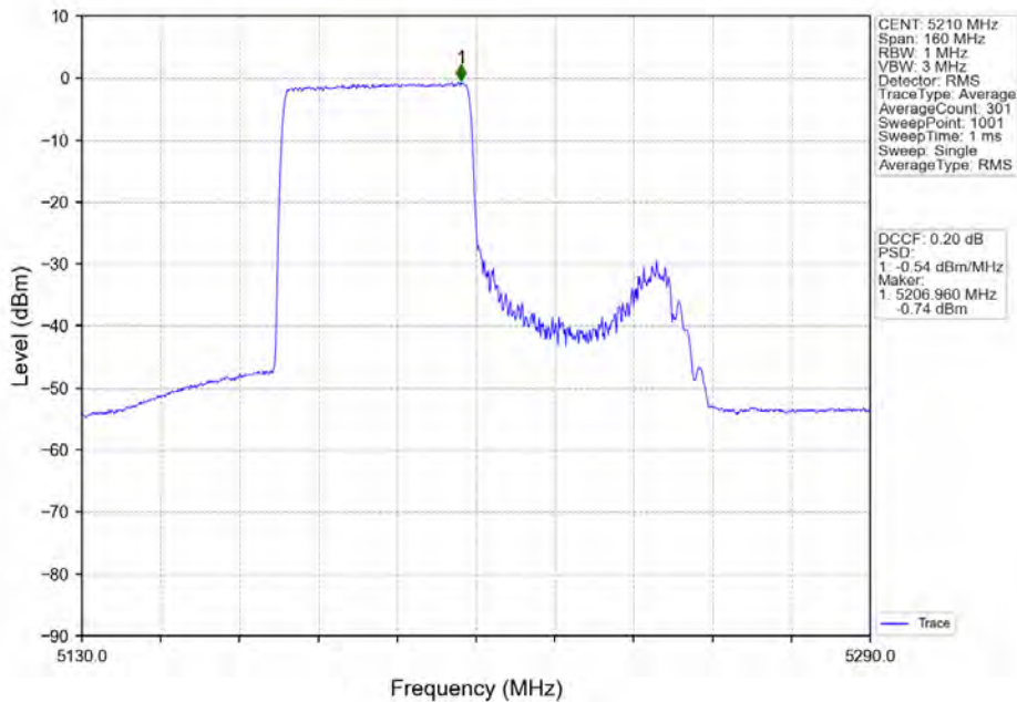
802.11ax(HE80)_MCH_5210MHz_RU484_Left_Ant1_NTNV
