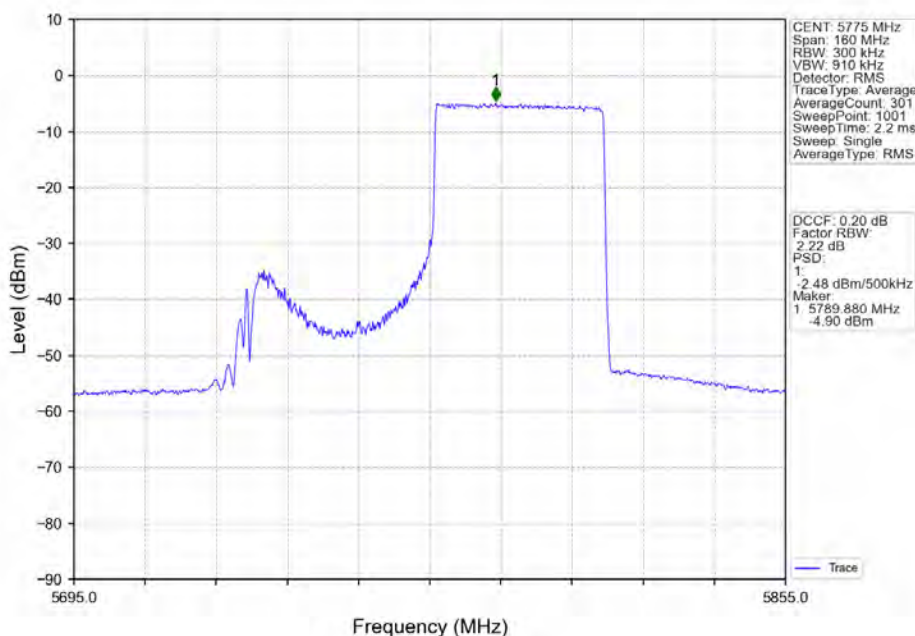
802.11ax(HE80)_MCH_5775MHz_RU484_Right_Ant1_NTNV
