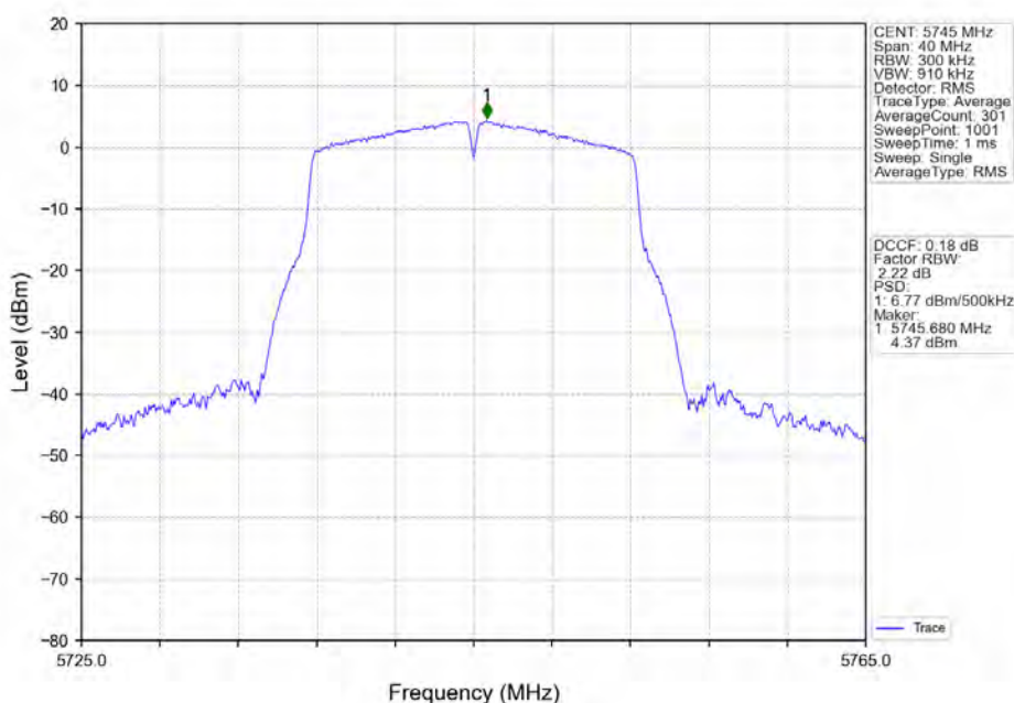
802.11a_LCH_5745MHz_Ant2_NTNV
