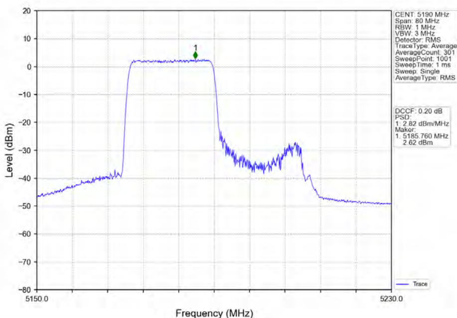
802.11ax(HE40)_LCH_5190MHz_RU242_Left_Ant2_NTNV
