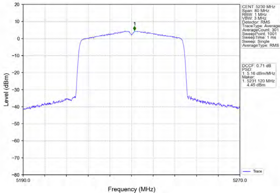
802.11ax(HE40)_HCH_5230MHz_RU484_Left_Ant2_NTNV
