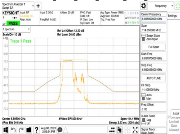
802.11be_20MHz_Chain1_6895MHz_RU26_0
