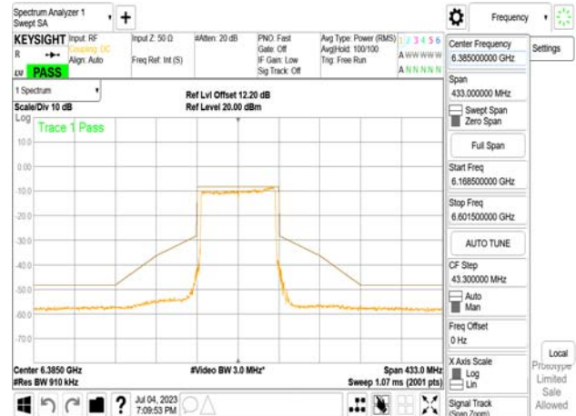
802.11be_80MHz_Chain0_6385MHz_RU484+242_Punc20
