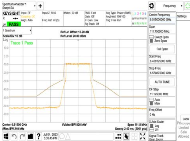
802.11be_20MHz_Chain1_6515MHz_106+26_MRUG
