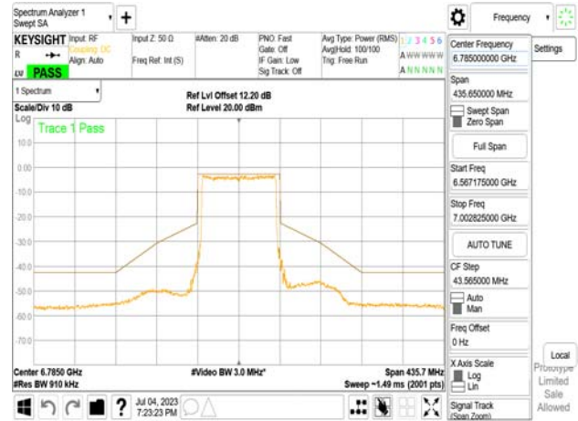
802.11be_80MHz_Chain1_6785MHz_RU484+242_Punc20
