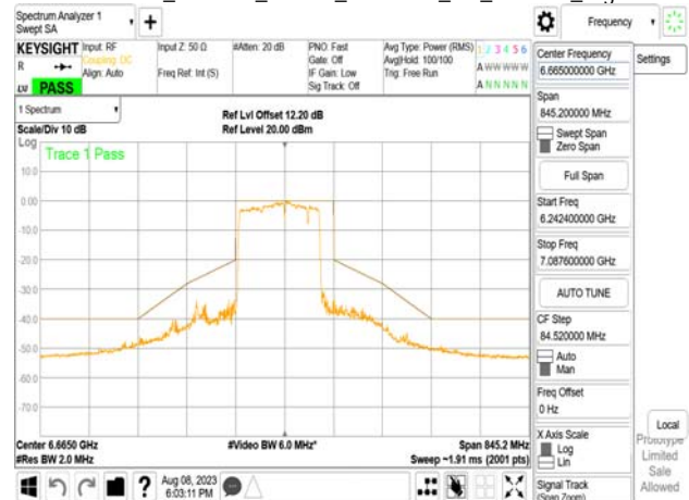
802.11be_160MHz_Chain1_6665MHz_SU_Punct20_Mid3
