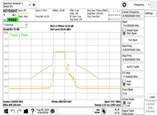
802.11be_20MHz_Chain1_6895MHz_52+26_MRUI
