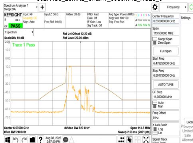
802.11be_20MHz_Chain1_6535MHz_RU26_0
