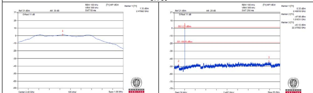
CH 0 Band edge
