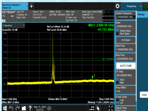
Band2-20MHz-QPSK-18700-1RB#0-1000~3000-PASS
