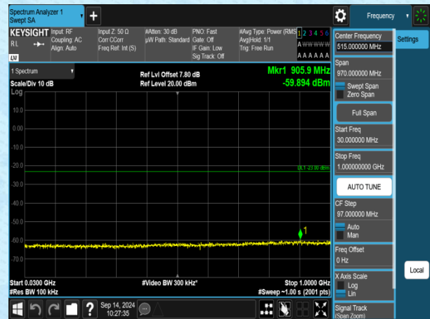
Band2-20MHz-QPSK-18700-1RB#0-30~1000-PASS
