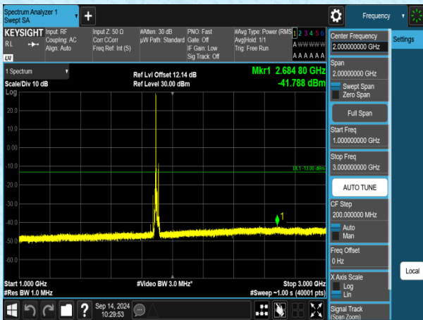
Band2-20MHz-QPSK-19100-1RB#0-1000~3000-PASS
