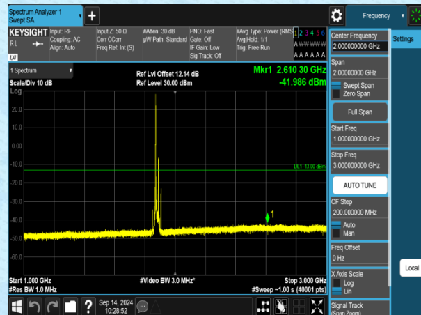
Band2-20MHz-QPSK-18900-1RB#0-1000~3000-PASS
